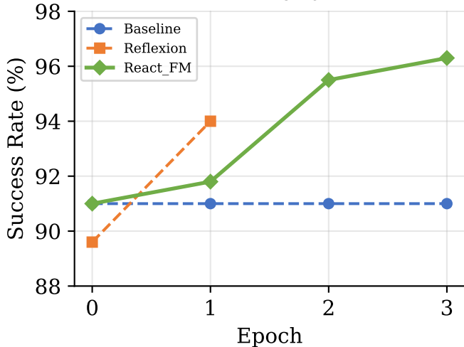
ALFWorld
