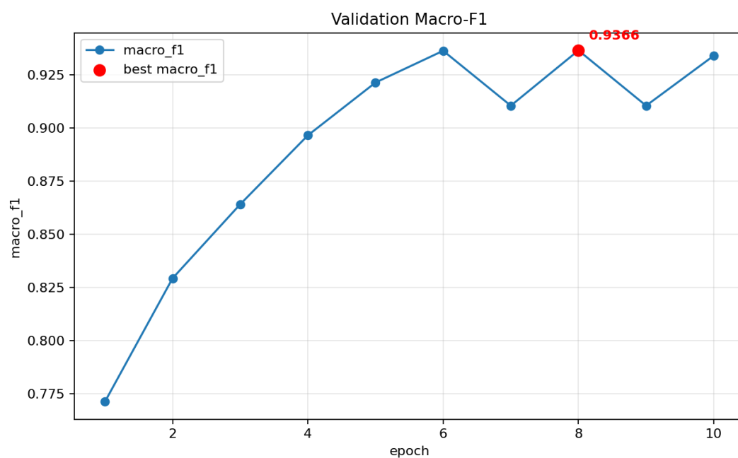
图 4: 验证集 Macro F1 随训练轮次变化曲线
