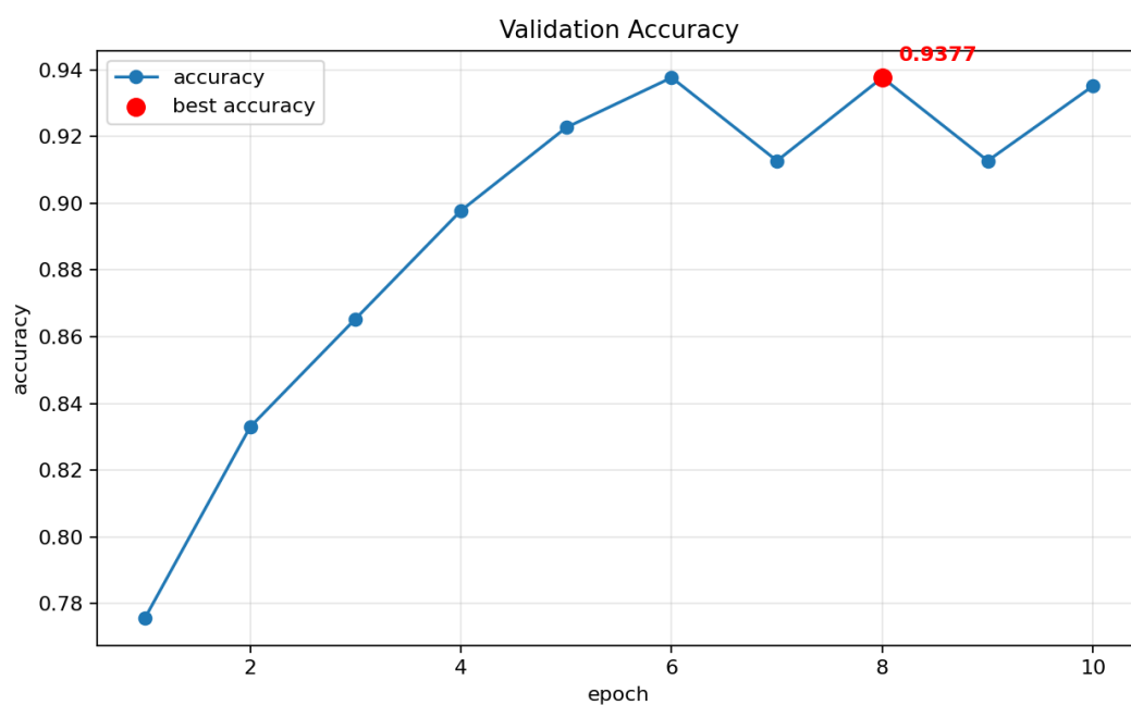
图 3: 验证集 Accuracy 随训练轮次变化曲线
