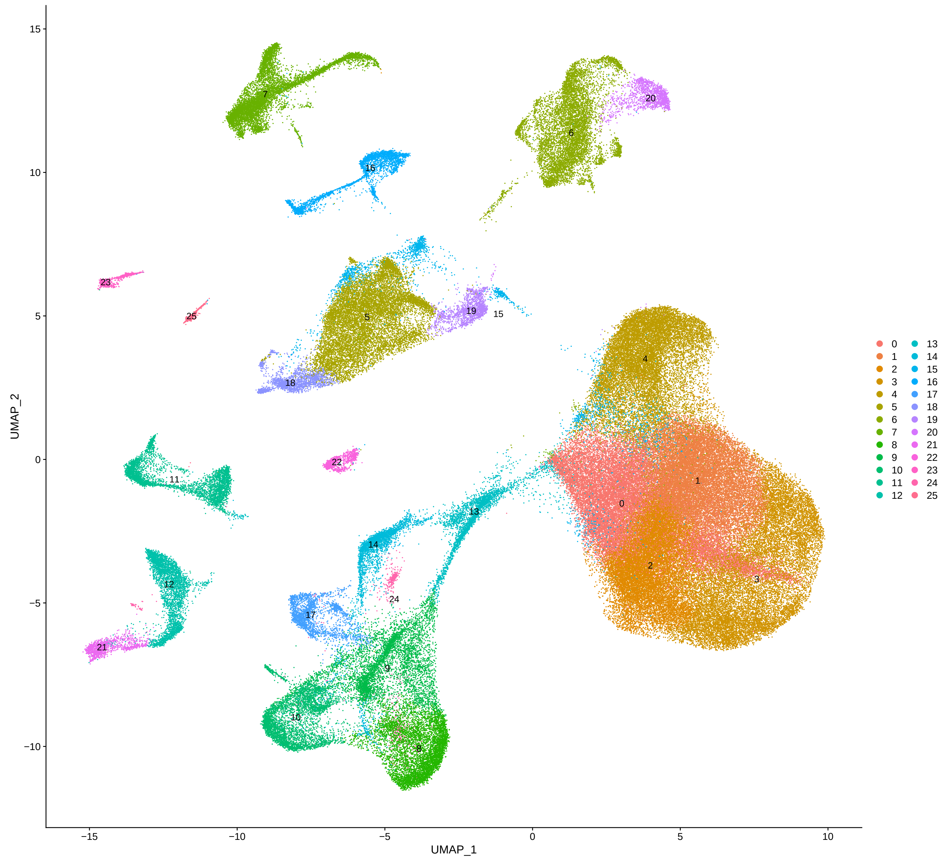
Lake_Jakel_Absinta_RRSP_Schirmer_seurat_clusters
