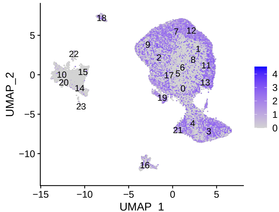
OLIG2
