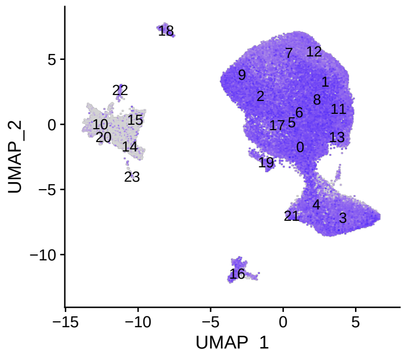
MAG
