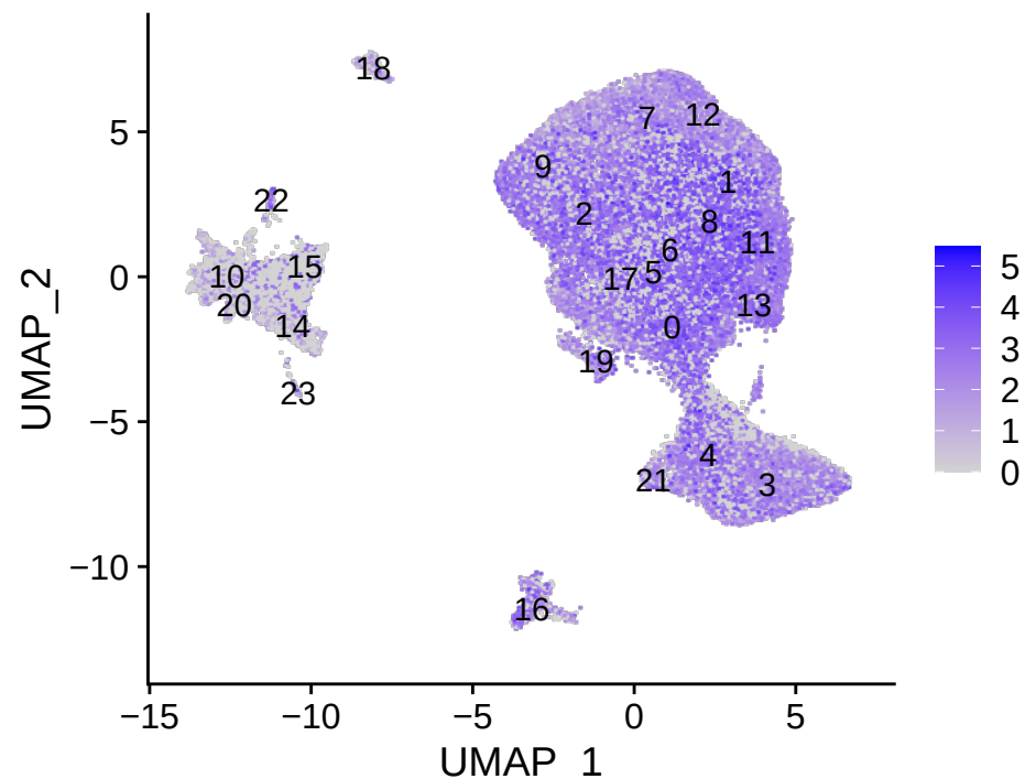
MOG
