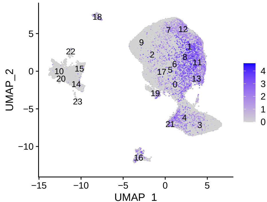
LINGO1
