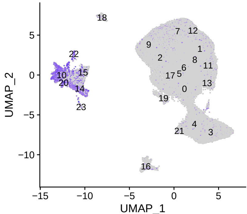
PDGFRA
