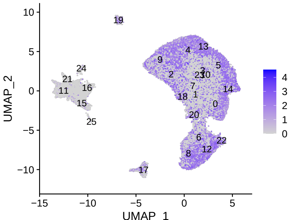
OLIG2
