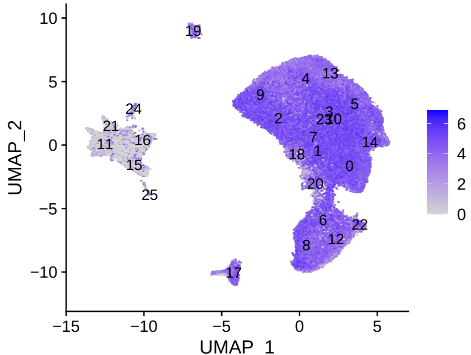
MAG
