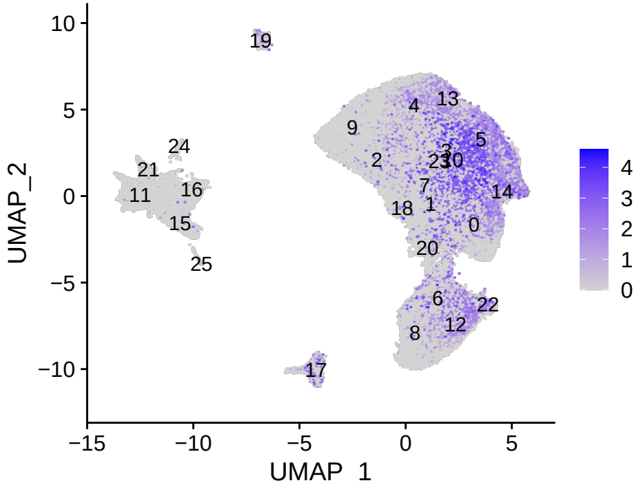
LINGO1
