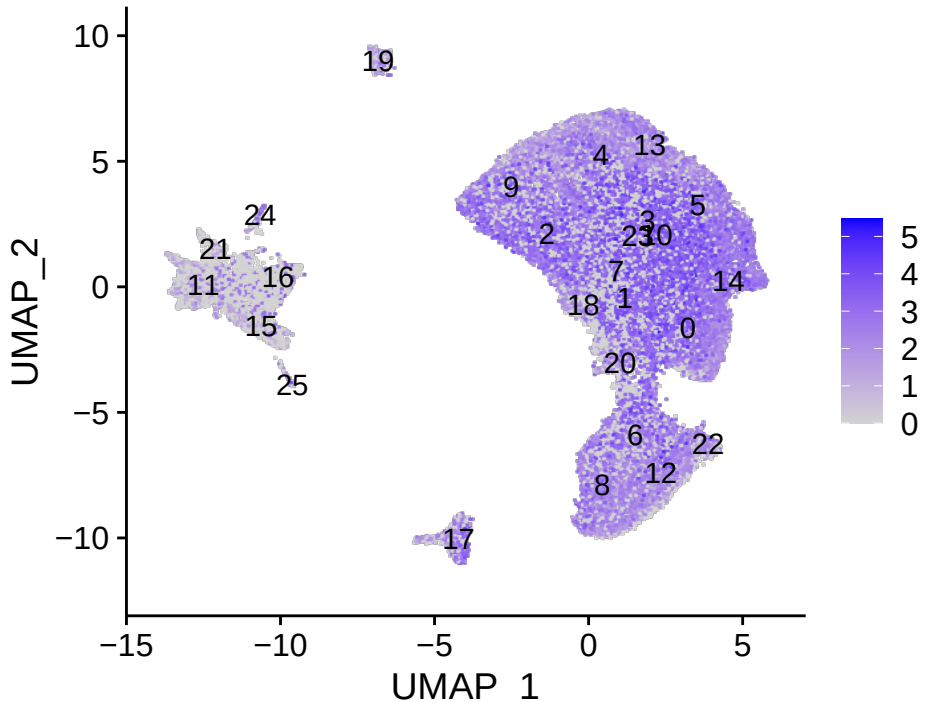
MOG
