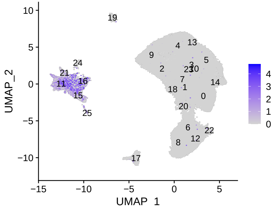
PDGFRA
