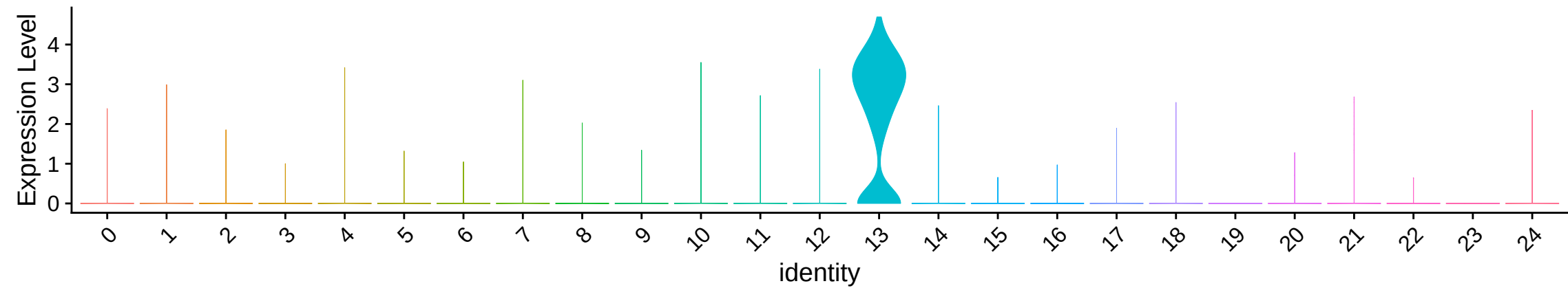
SKAP1
