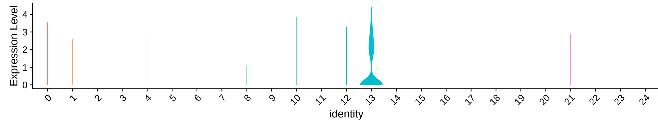
CCL5
