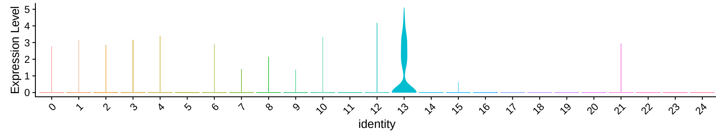
CD4
