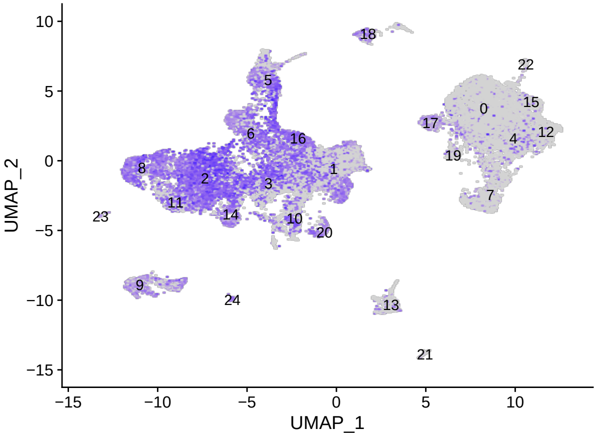
VIM
