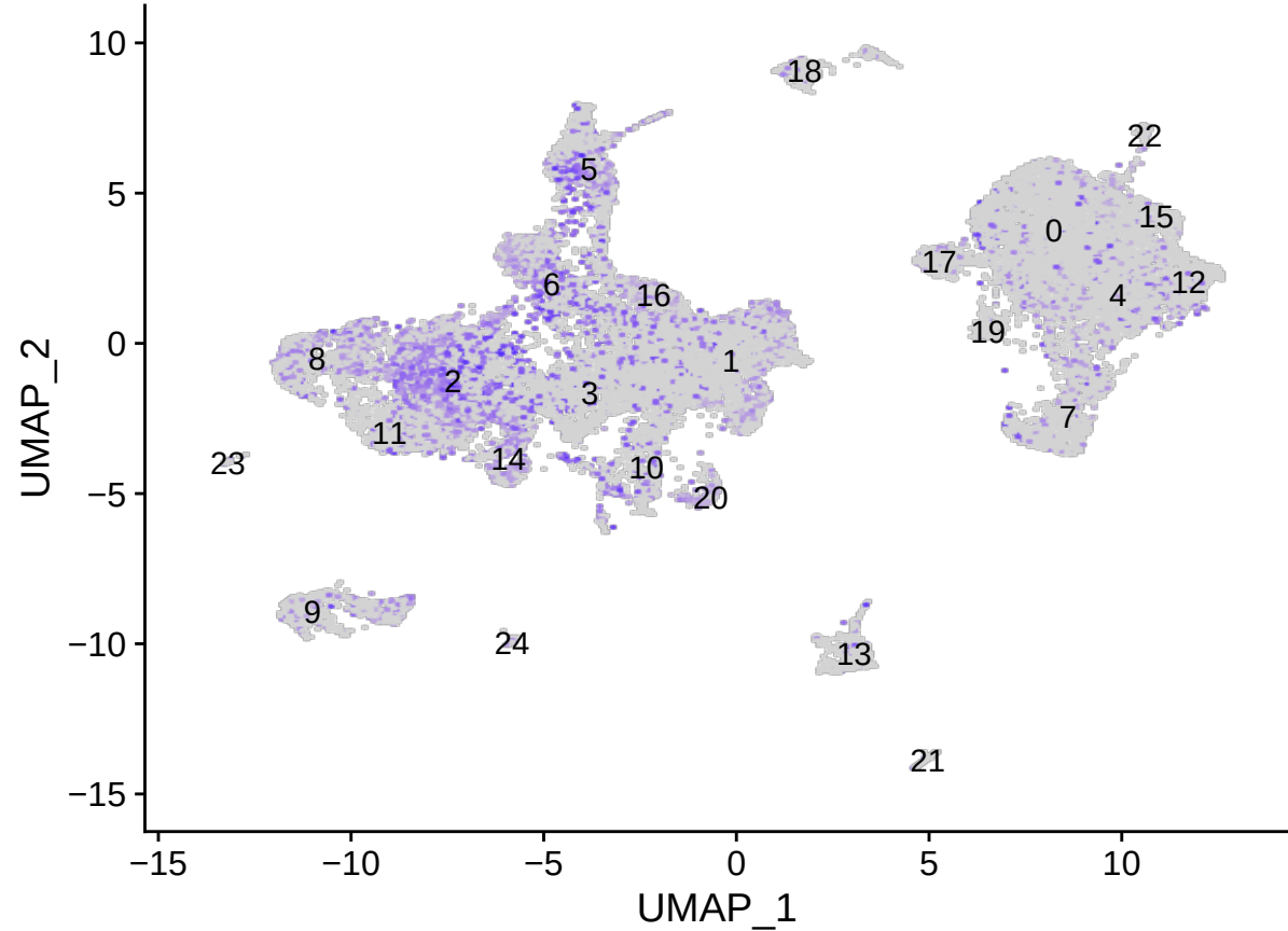
FTL
