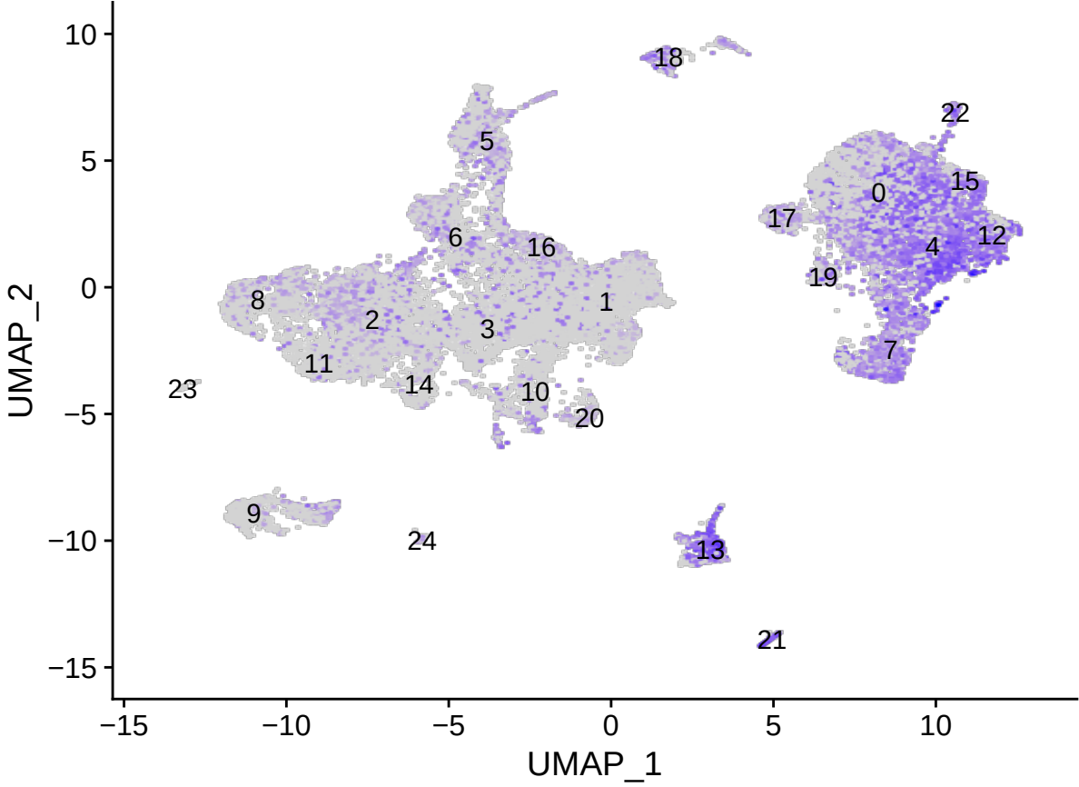
B2M
