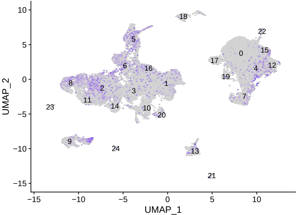
SOD1
