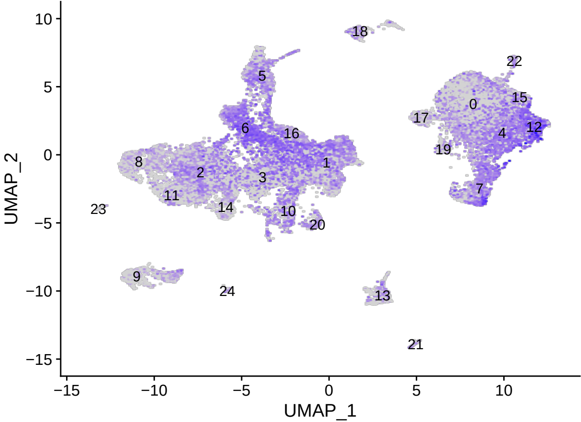
B2M
