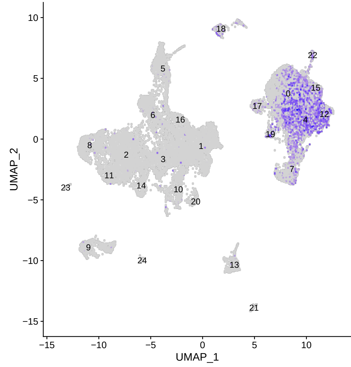
IL1B
