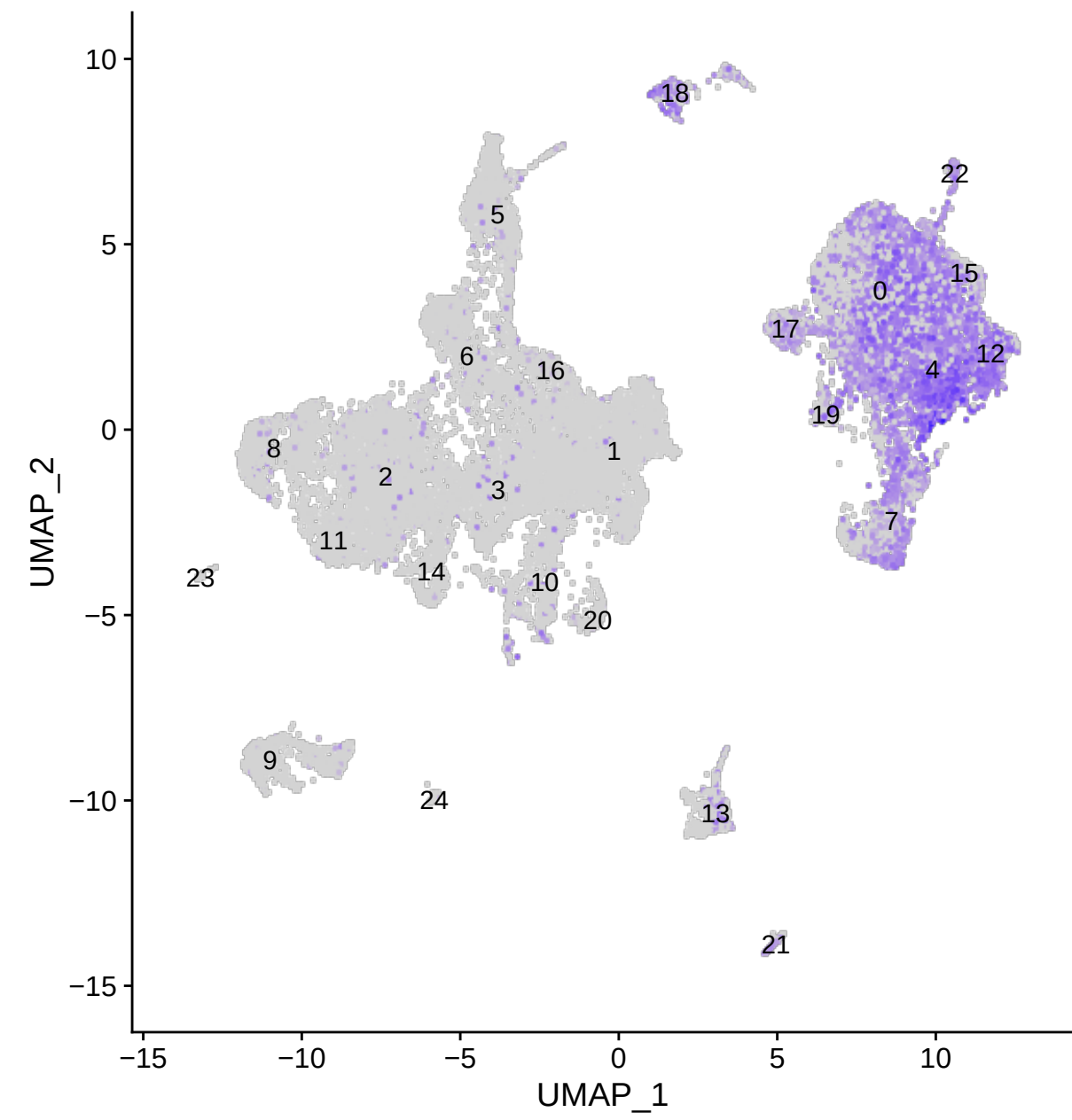
C1QA
