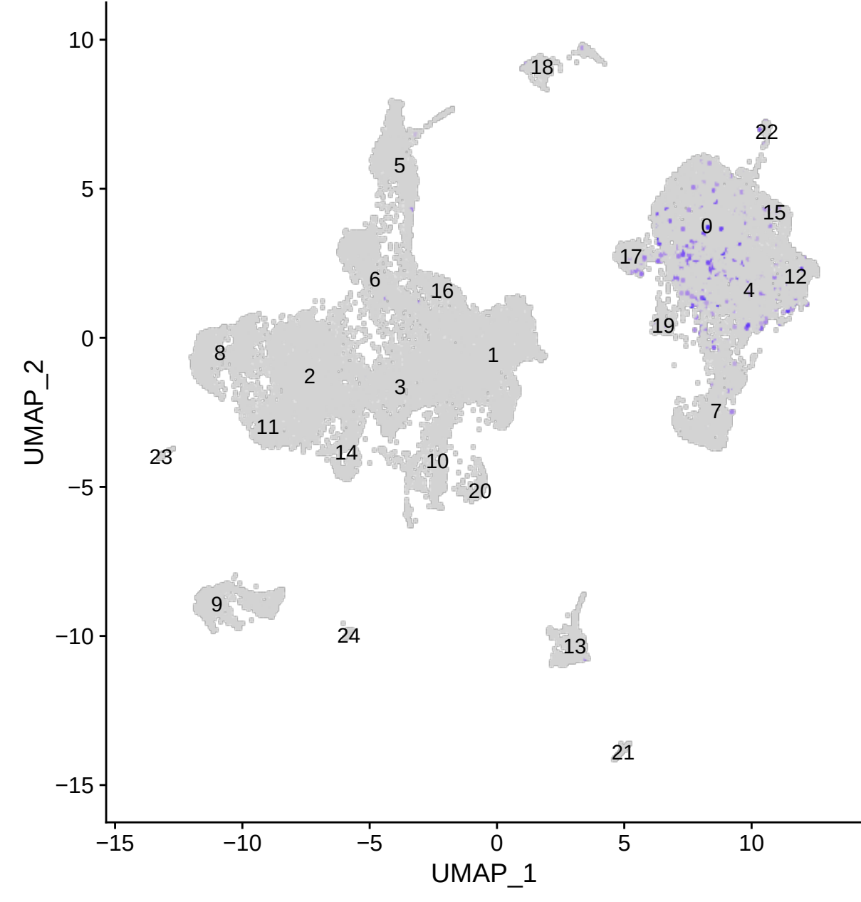
IL1B
