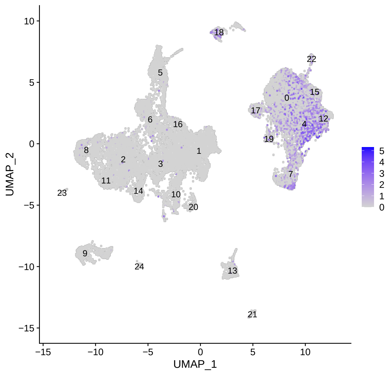
SOD1
