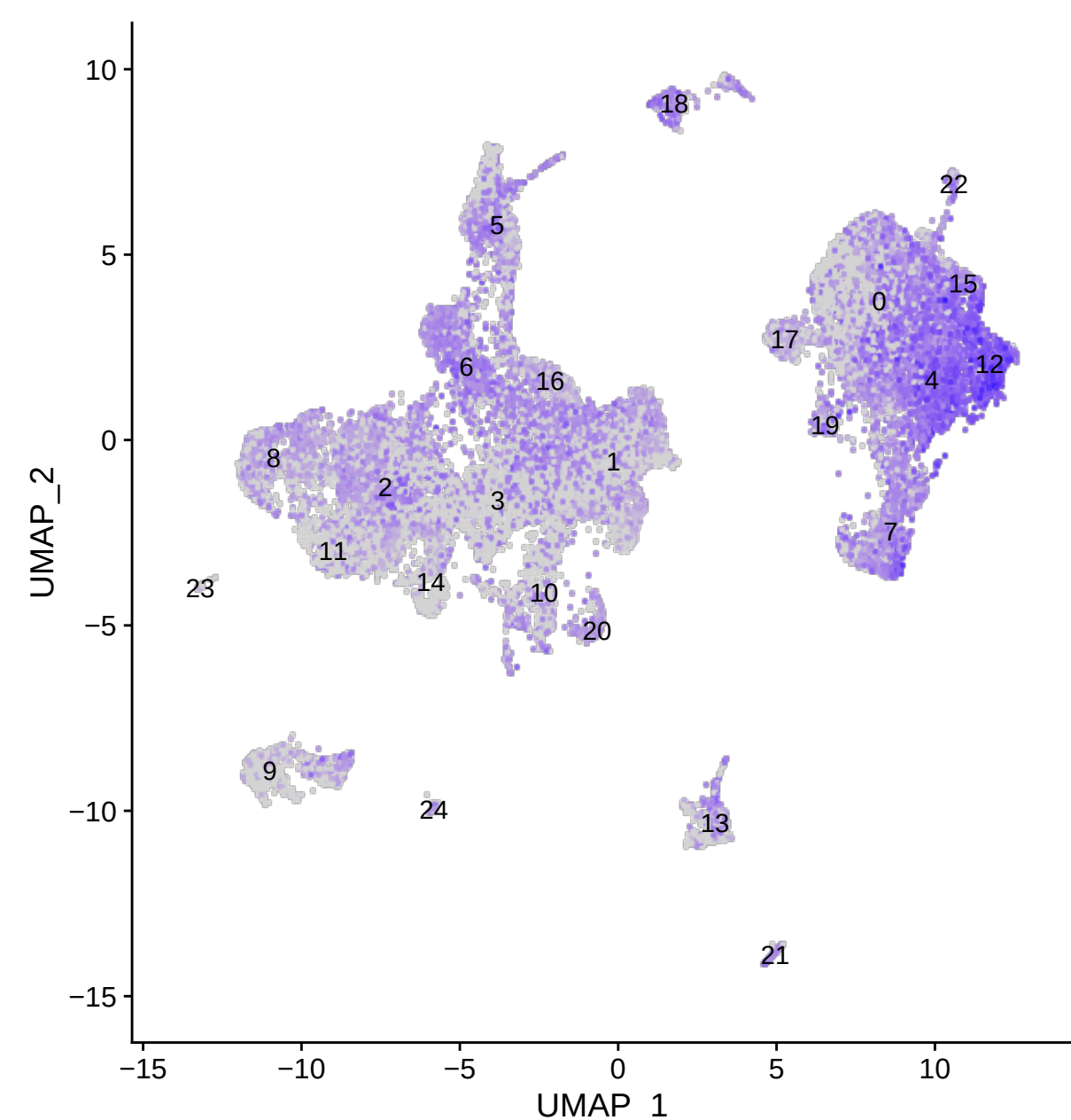
HLA-DRA
