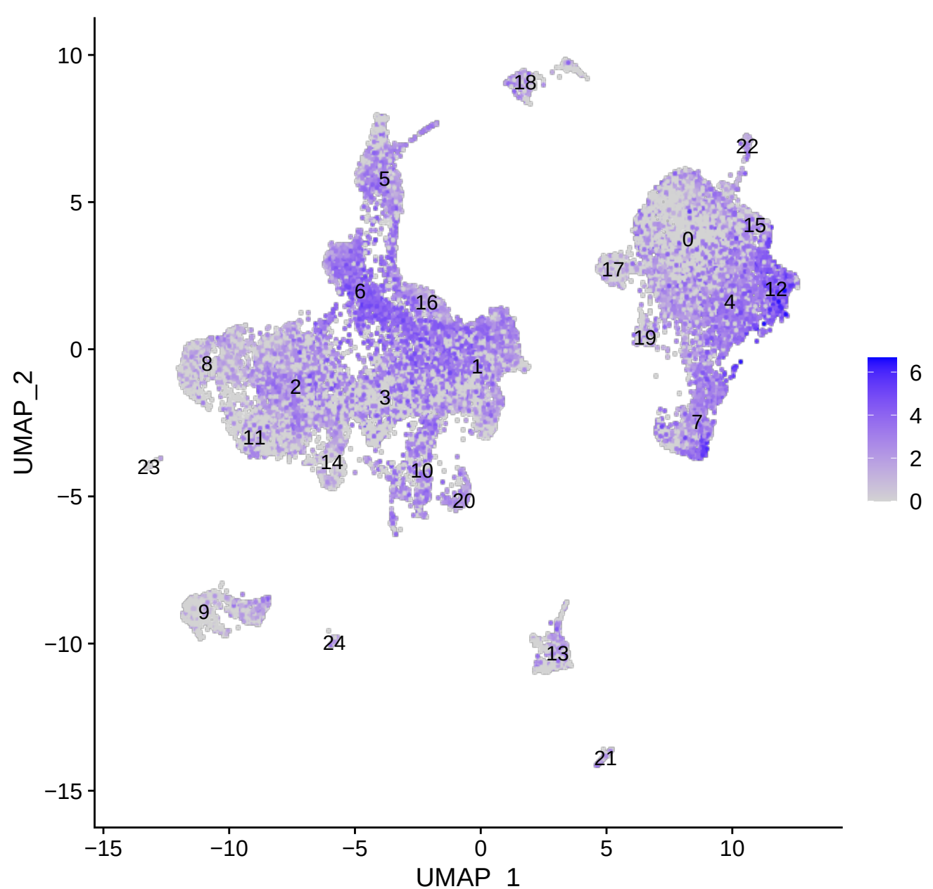
HLA-DPA1
