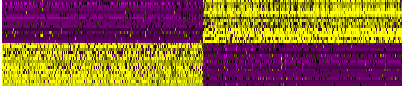
PC_6
