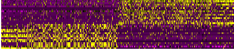
PC_15
