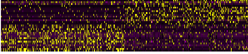
PC_29
