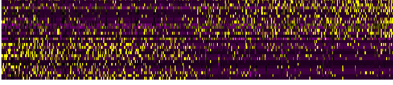
PC_37
