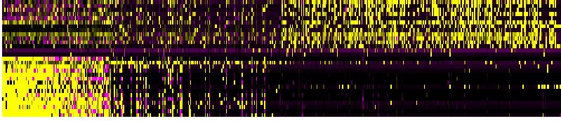
PC_22
