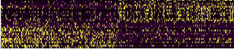
PC_35
