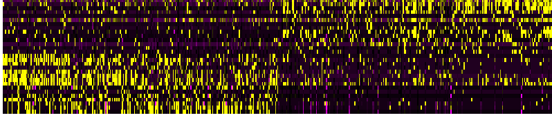
PC_36
