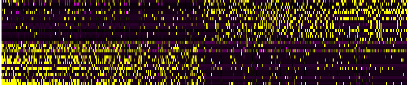
PC_26
