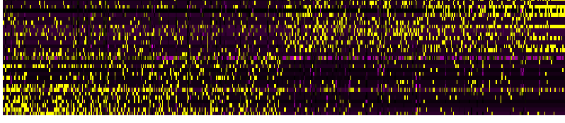
PC_39
