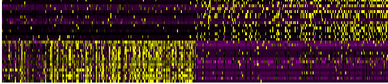
PC_12
