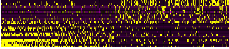
PC_25
