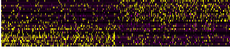
PC_45
