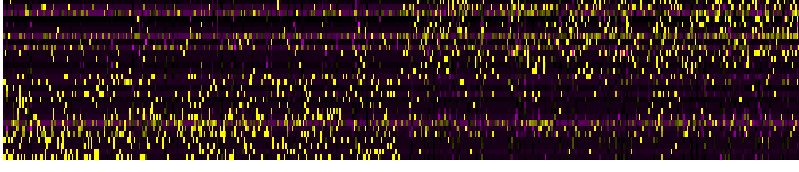
PC_46
