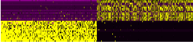
PC_7
