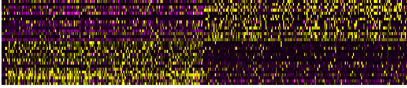
PC_23
