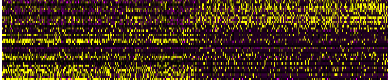
PC_30
