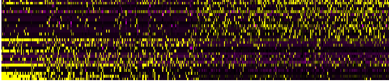
PC_32
