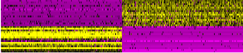
PC_4
