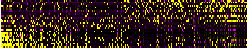
PC_50
