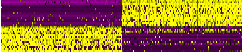
PC_9
