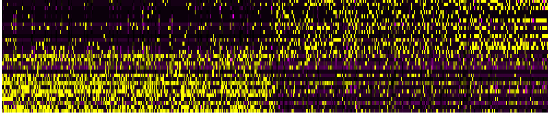
PC_31
