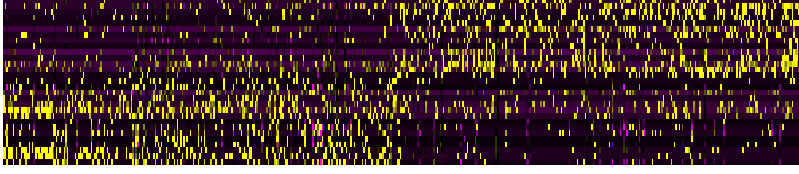
PC_34
