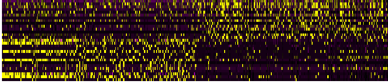
PC_27
