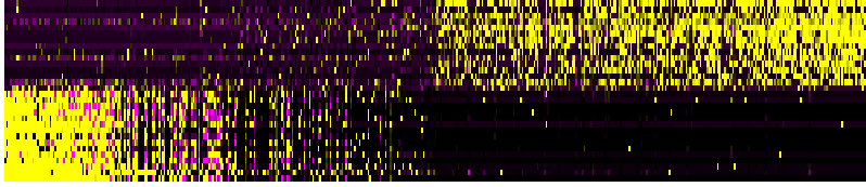
PC_21
