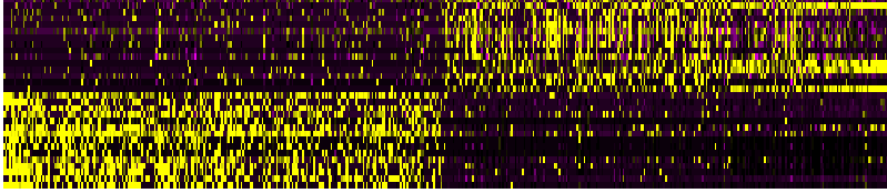
PC_17
