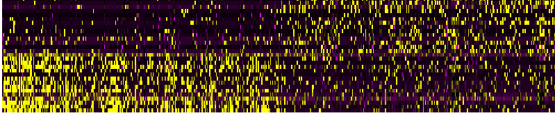
PC_38
