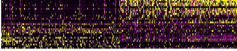
PC_33
