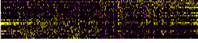
PC_49
