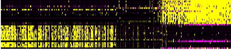
PC_13
