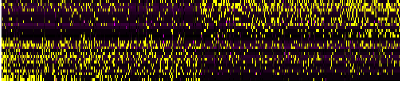
PC_44
