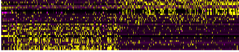
PC_24
