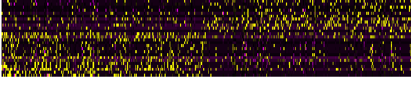
PC_49
