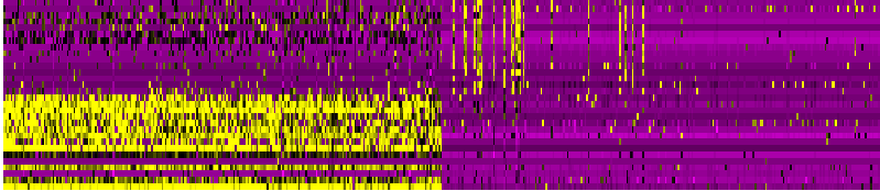
PC_8
