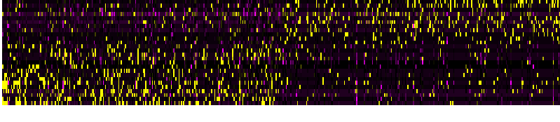
PC_50
