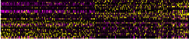
PC_40
