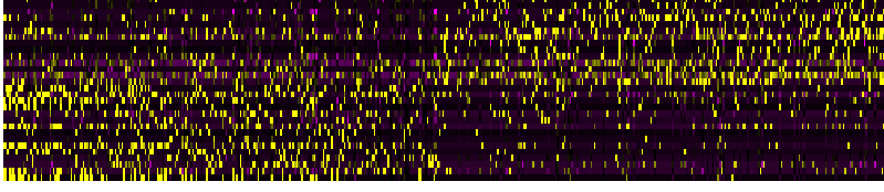
PC_41
