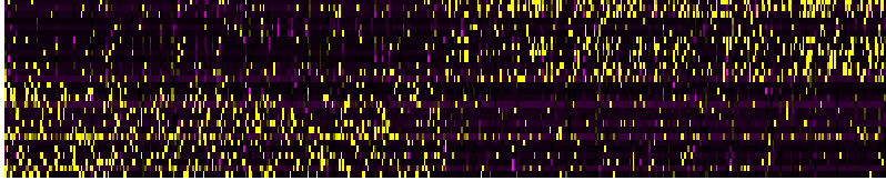
PC_48
