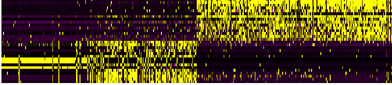
PC_14
