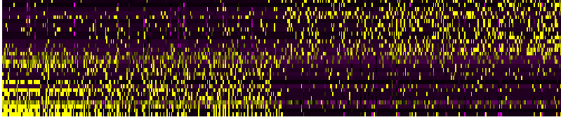
PC_28
