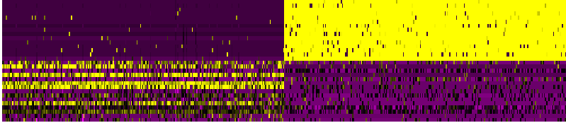
PC_5
