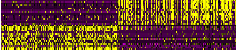
PC_11
