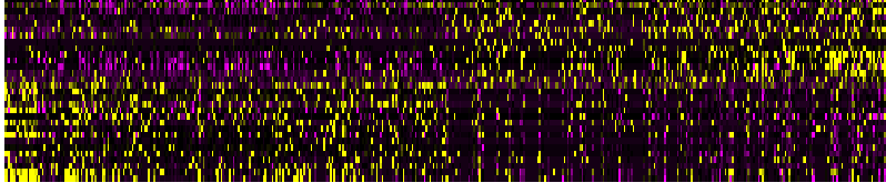
PC_42
