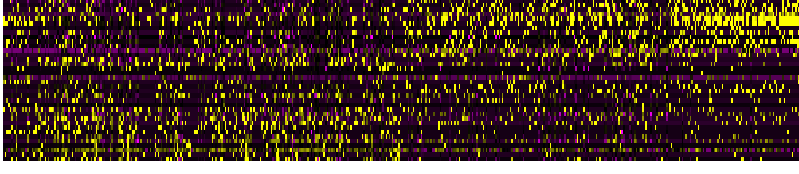
PC_43
