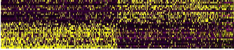
PC_20
