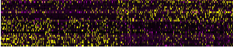
PC_47
