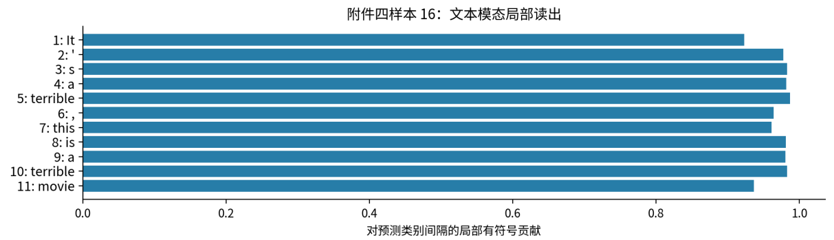
图 5.6 附件 4 样本 16 的主要参考模态内局部重要性。每行给出原 BERT 位置和对应原文，负值表示反对当前类别间隔；词的上下文由 BERT 编码。
