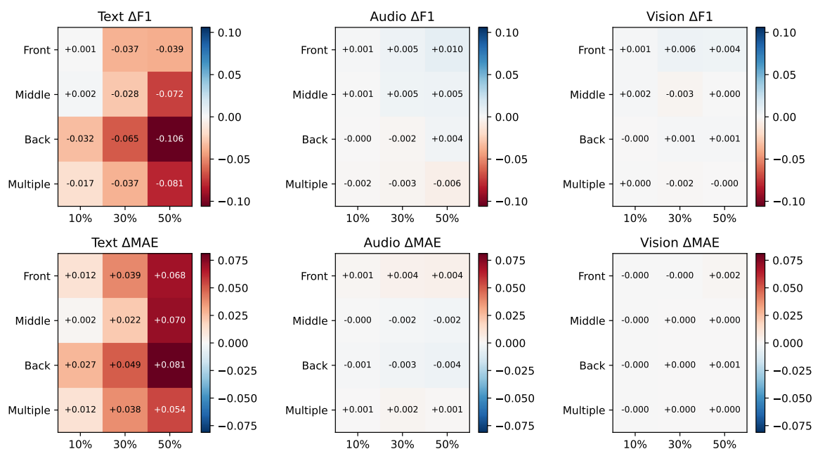
图 4.3 定版模型的 36 类位置与形状对照。上排为相对完整输入的 F1 变化，下排为 MAE 变化；同一指标共用色标。
