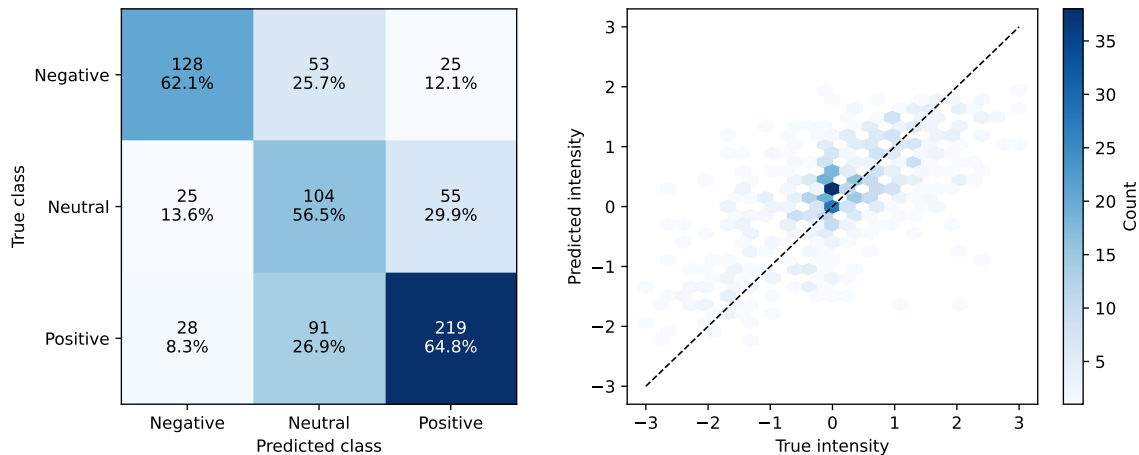
图 4.4 定版模型在 728 条验证样本上的错误分析。左图为混淆矩阵，格内显示计数及真实类别内比例；右图为真实强度与预测强度的二维计数，虚线表示理想预测。
