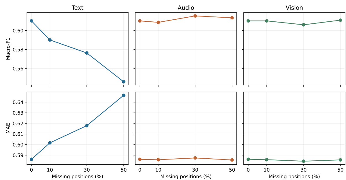
图 4.2 定版模型在官方验证集的连续缺失比例响应。0% 为完整输入；横轴表示有效特征位置中的名义缺失比例。各行共用纵轴，F1 越高越好，MAE 越低越好。
