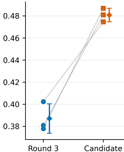
(c) Neutral F1
