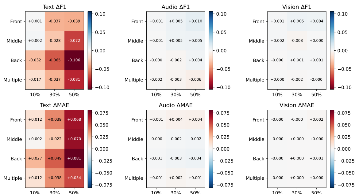
图 4.3 最终模型的 36 类位置与形状对照。上排为相对完整输入的 F1 变化，下排为 MAE 变化；同一指标共用色标。
