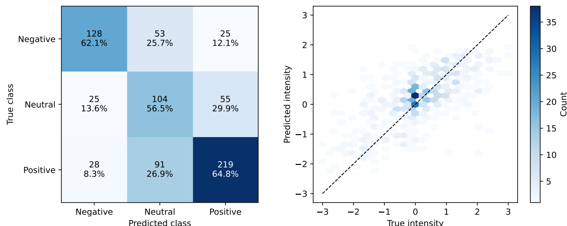
图 4.4 最终模型在 728 条验证样本上的错误分析。左图为混淆矩阵，格内显示计数及真实类别内比例；右图为真实强度与预测强度的二维计数，虚线表示理想预测。
