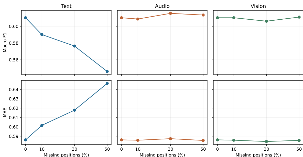
图 4.2 最终模型在验证集的连续缺失比例响应。0% 为完整输入；横轴表示有效特征位置中的名义缺失比例。各行共用纵轴，F1 越高越好，MAE 越低越好。
