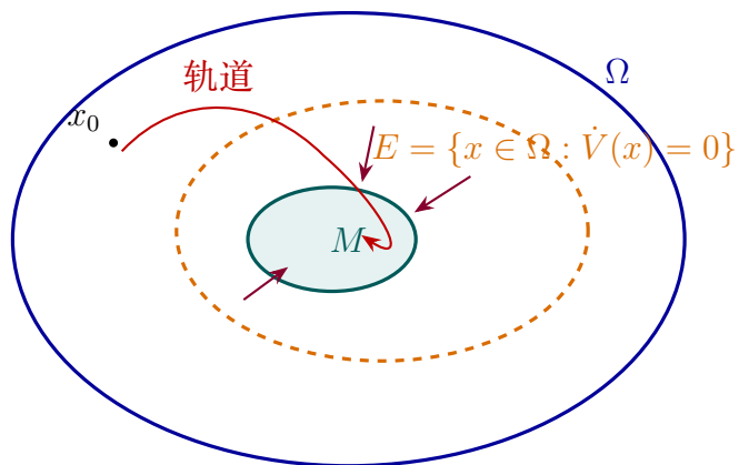
图 2.6: LaSalle 不变集原理示意图
