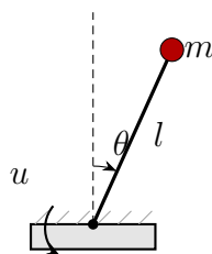
图 3.10: 固定支点倒立摆系统示意图。
