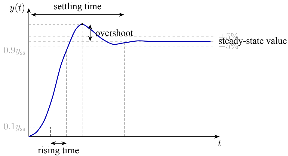
图 3.2: 典型阶跃响应中的 overshoot、rising time、settling time 与 steady-state value。
