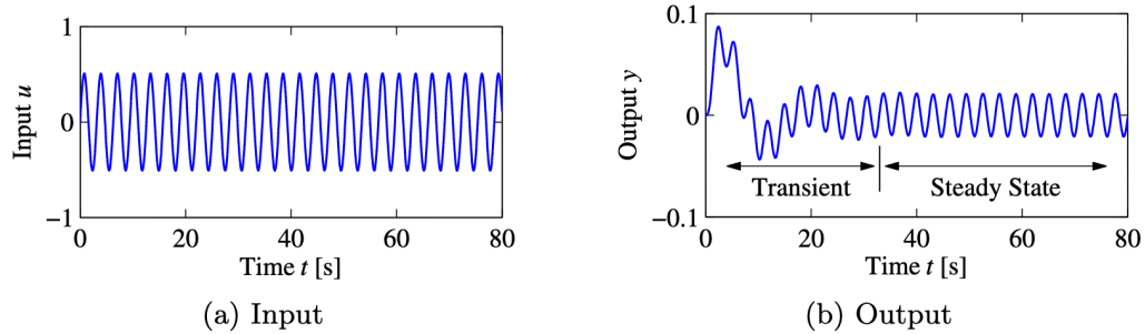
图 3.1: 瞬态响应与稳态响应 (Åström et al. 2021, Figure 6.8)
