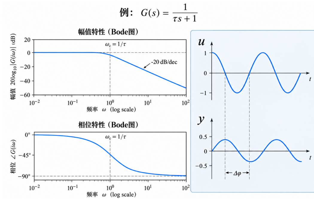
图 3.3: Bode 图示意图
