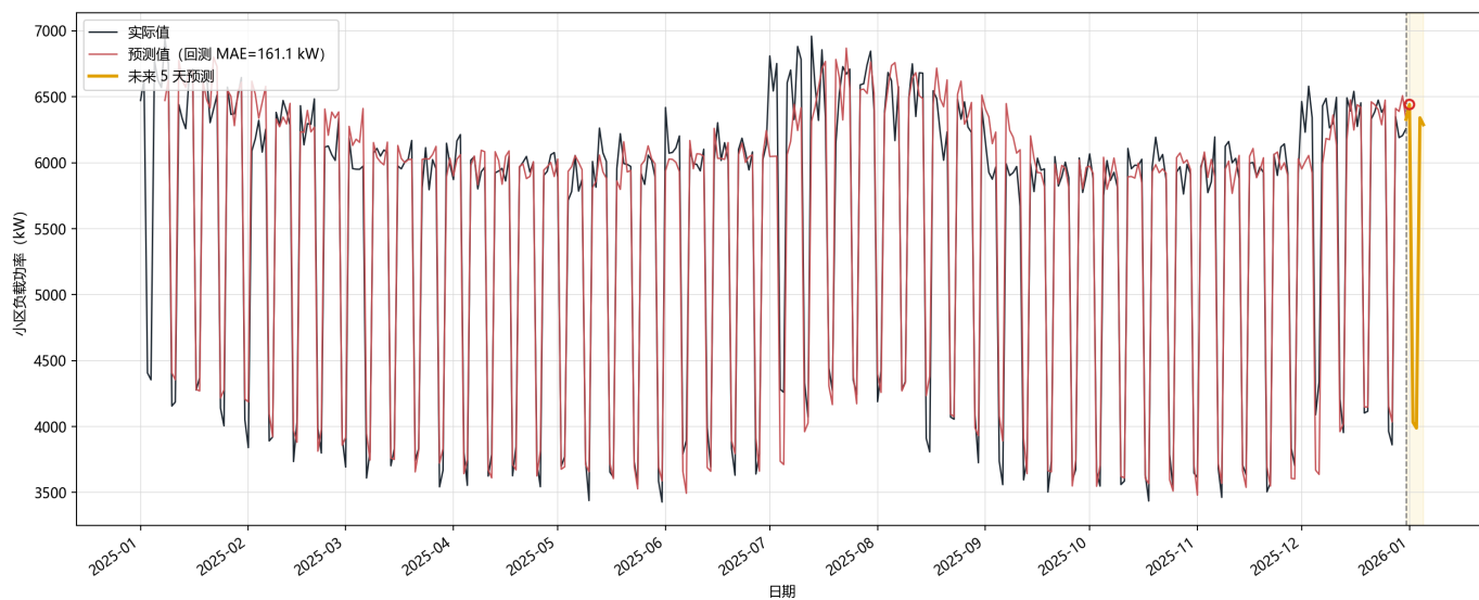
小区负载实际值与预测值对比 (每天 12:00)
