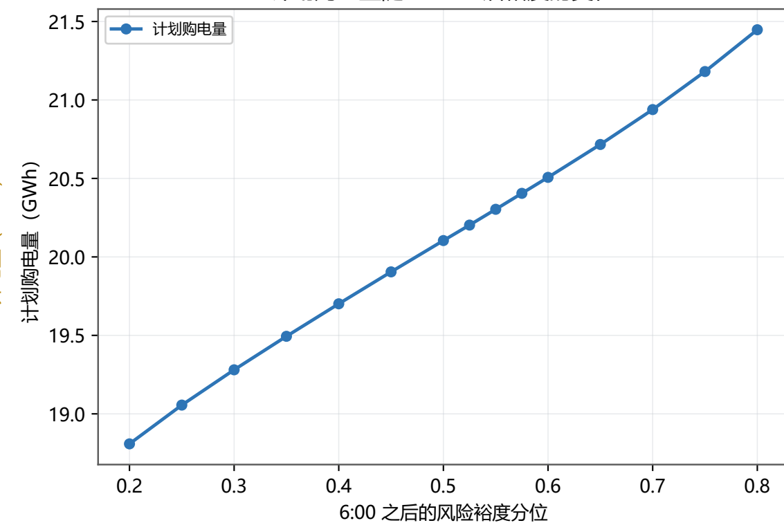
计划购电量随 6:00 之后裕度的变化
