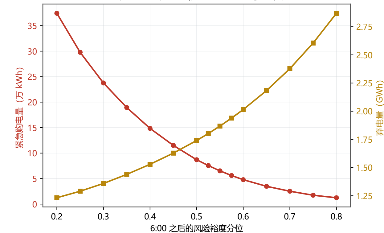
紧急购电量与弃电量随 6:00 之后裕度的变化
