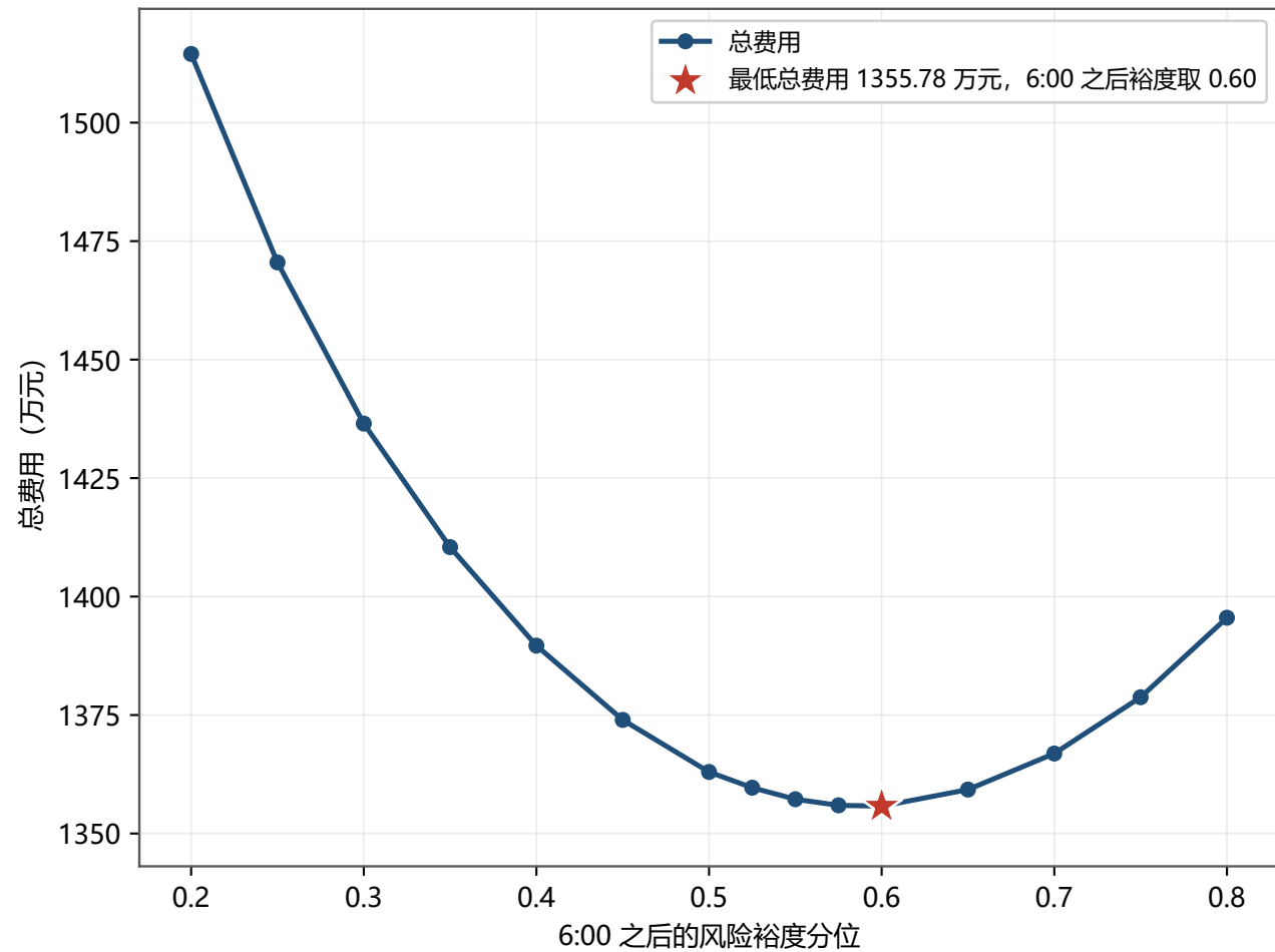
总费用随 6:00 之后裕度的变化, 0:00-6:00 裕度取 0.60
