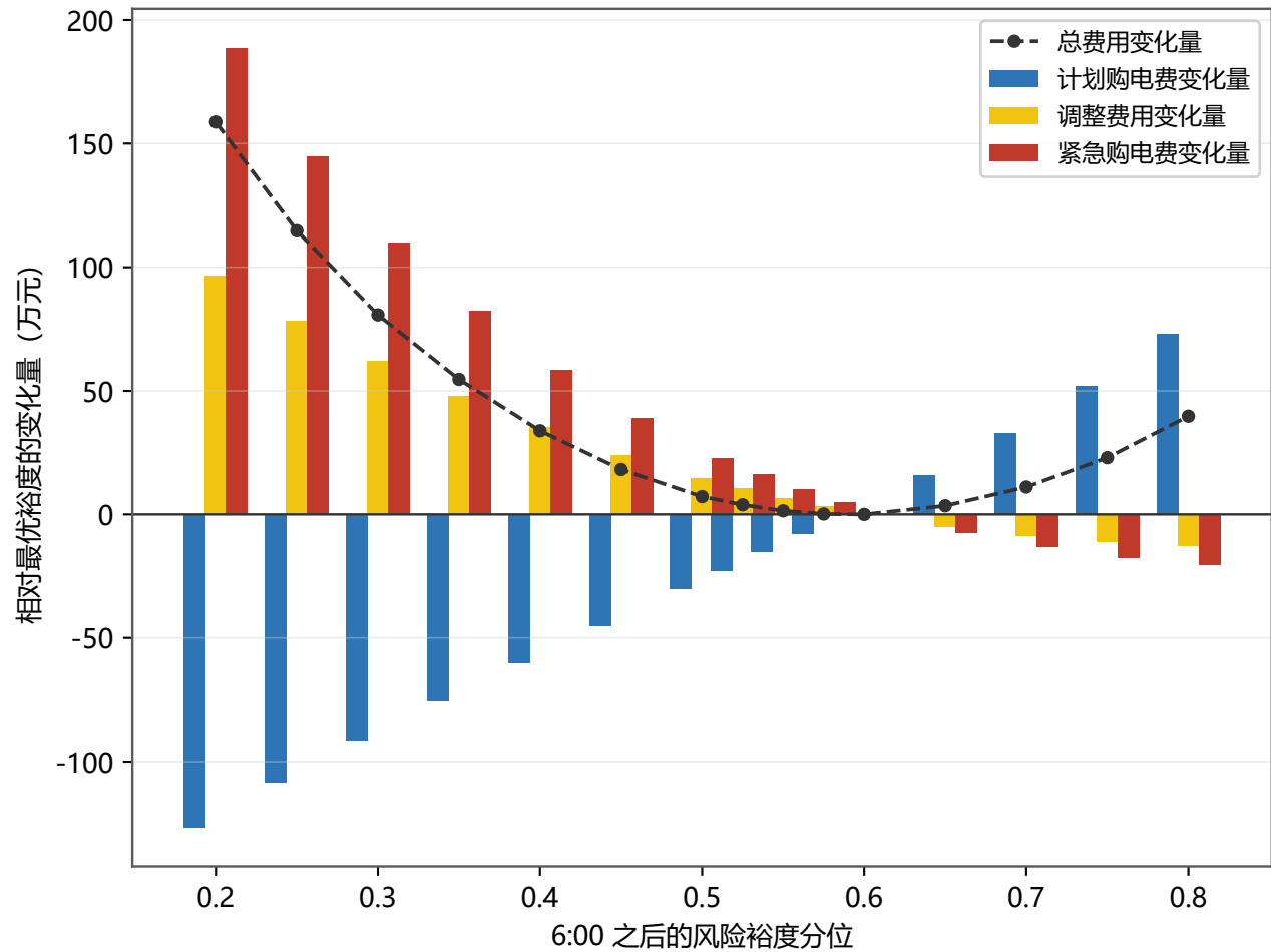
各费用项相对最优裕度的变化量
