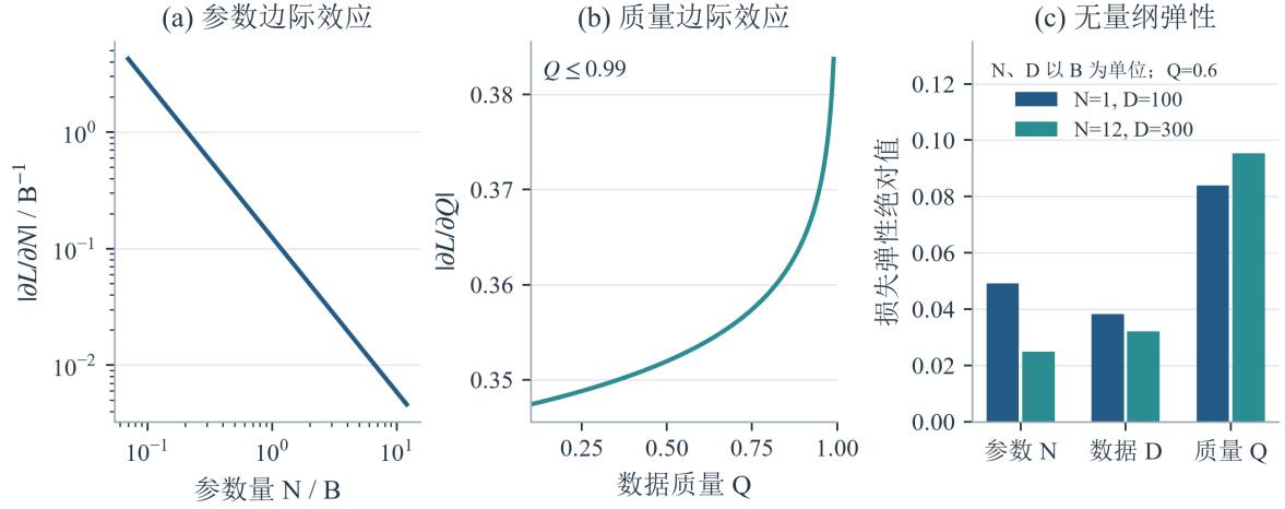
图 14 参数与质量的边际效应及参考点弹性
