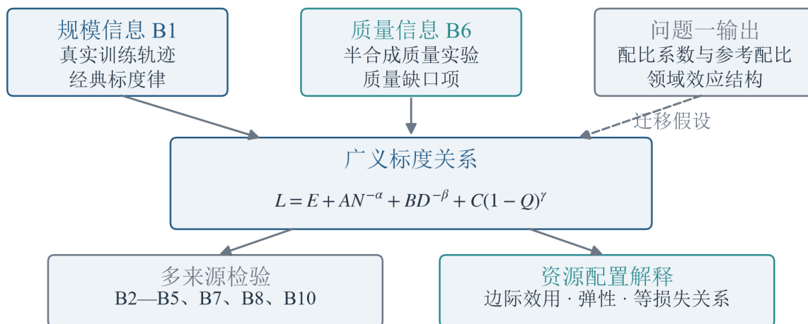
图9 规模、质量与领域效应的分析框架
