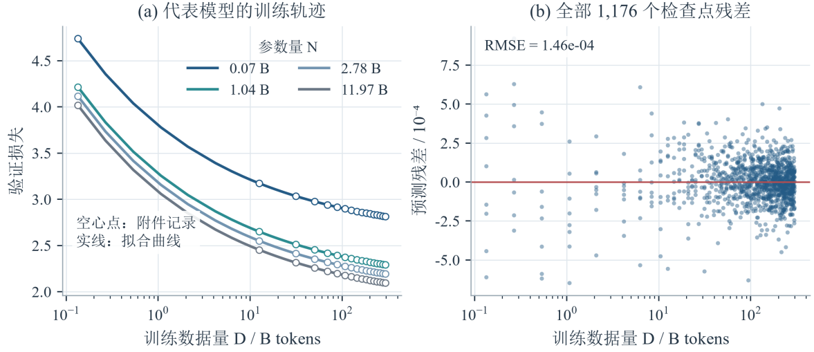
图 11 Pythia 代表模型的训练轨迹与全量拟合残差
