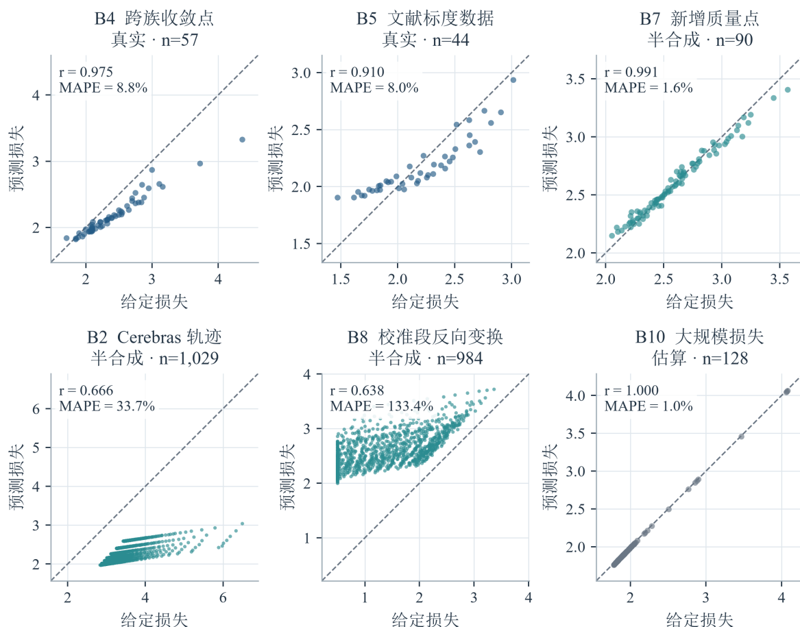
图 13 广义标度律在不同来源数据上的预测表现
