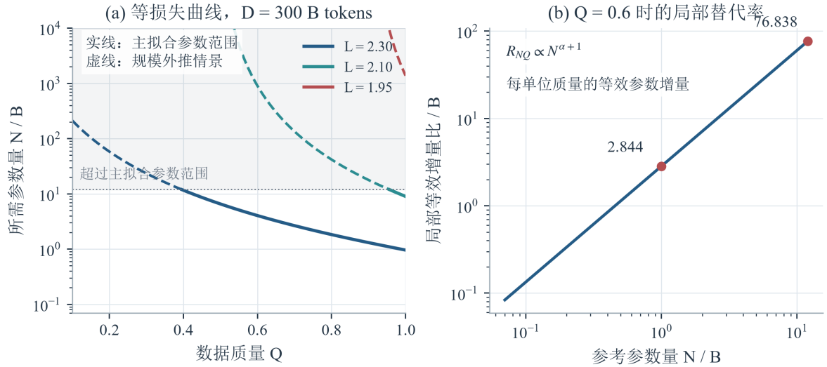
图 15 质量与参数规模的等损失关系及局部替代率
