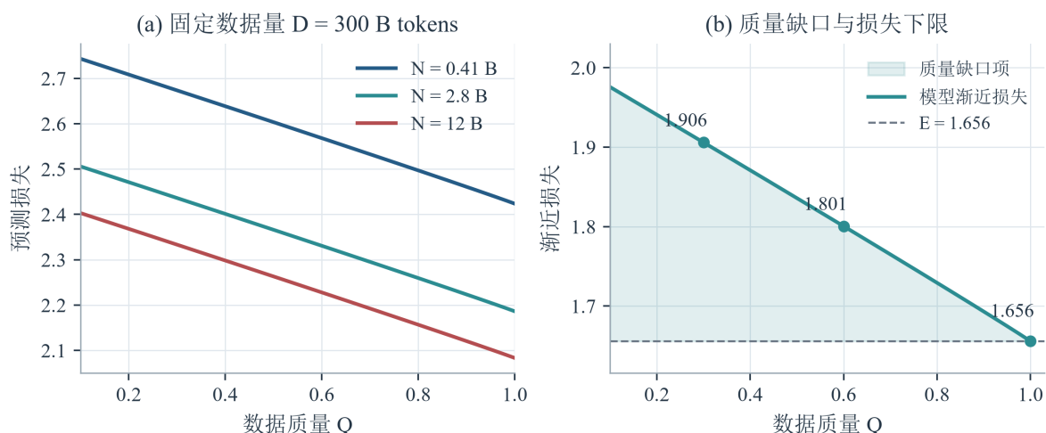
图 12 固定数据量下的质量效应与模型渐近损失
