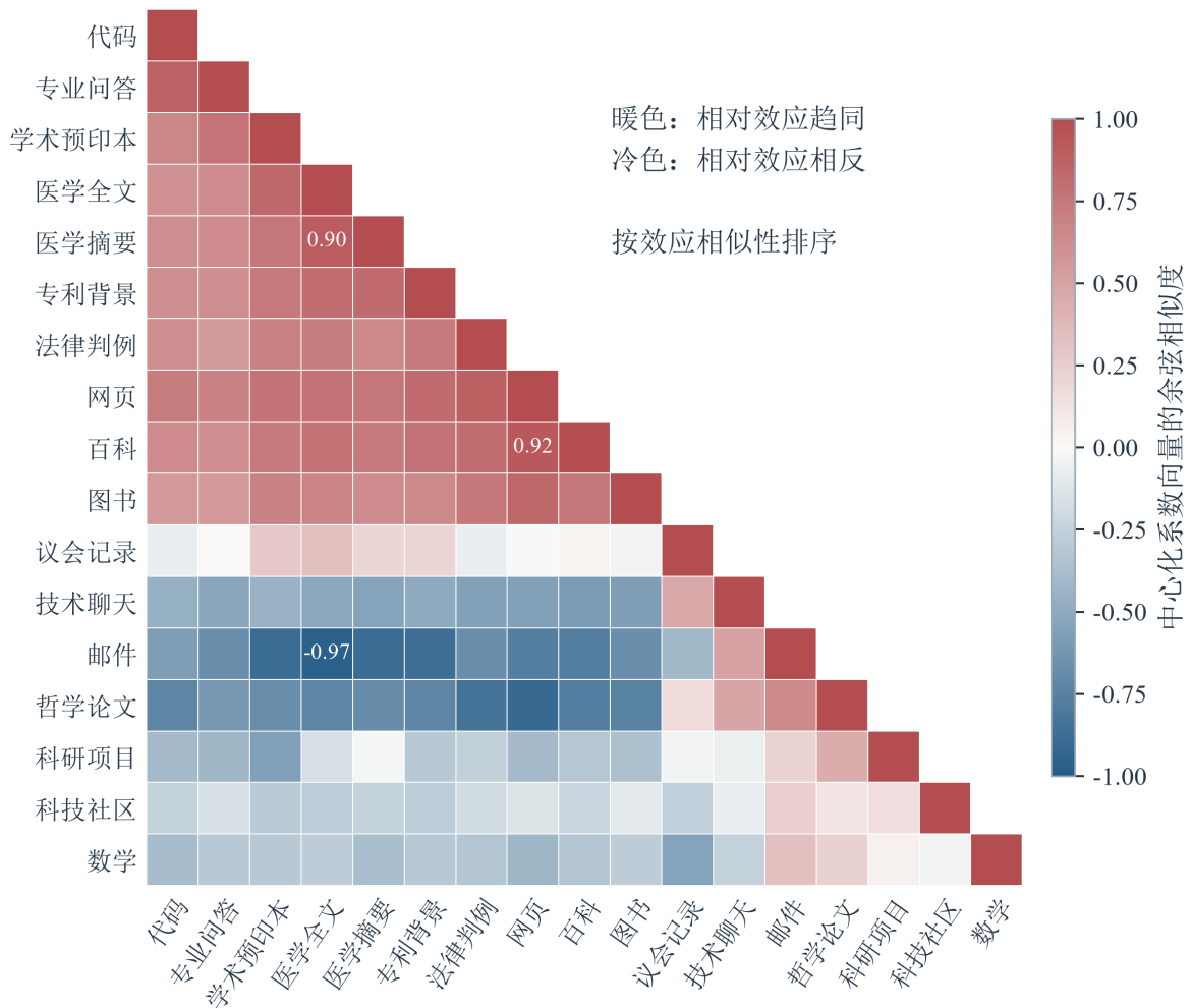
图 16 训练领域相对效应的余弦相似度
