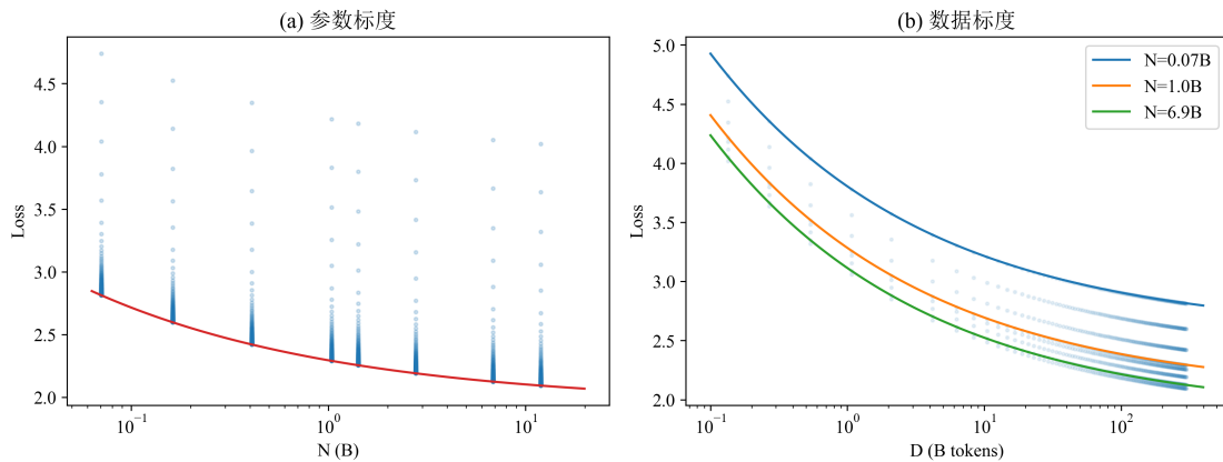
图 11 经典标度律对 Pythia 训练轨迹的拟合（左：随参数规模；右：随数据规模）
