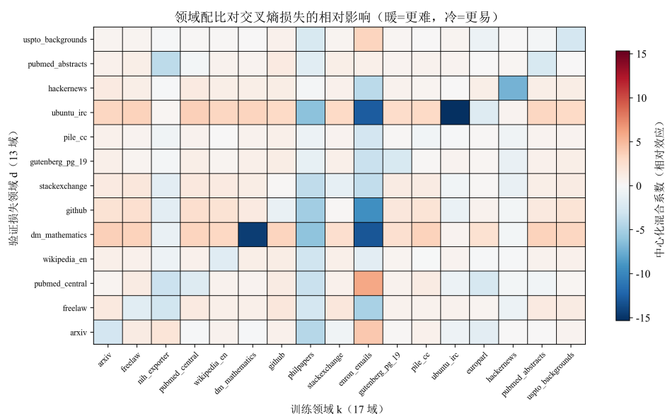
图 7 领域配比对交叉熵损失的相对影响热力图
