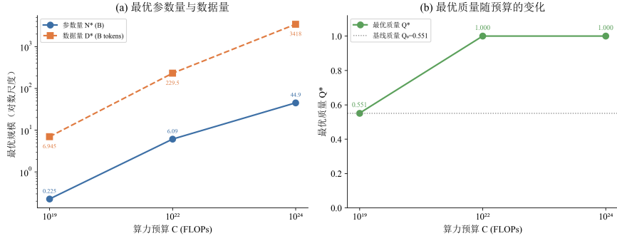
图 15 三档算力预算下的最优资源配置 ( N^* 、 D^* 、 Q^* )
