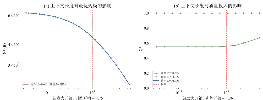
图 18 上下文长度敏感性 (左: 注意力开销对最优规模的影响; 右: 对质量投入的影响)
