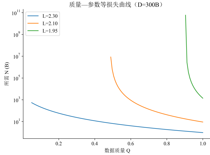
图 13 等损失曲线：达到同一损失所需参数量随质量的演化 ( D = 300B )
