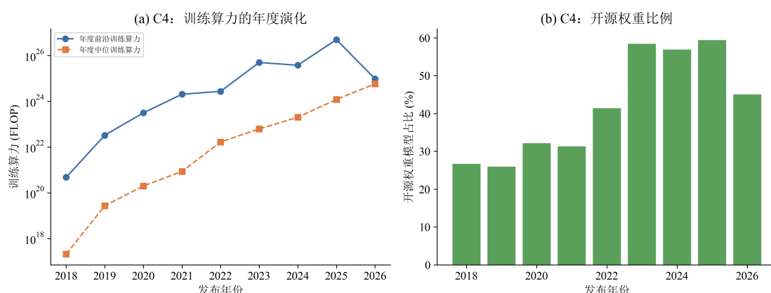
图 23 C4 宏观证据（左：训练算力的年度演化；右：开源权重模型占比）
