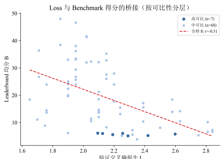
图 19 验证损失与 Leaderboard 均分的映射关系（按可比性分层）
