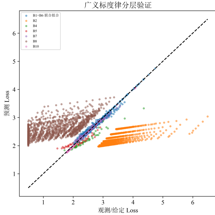
图 11 广义标度律预测值与实测损失的多源对比
