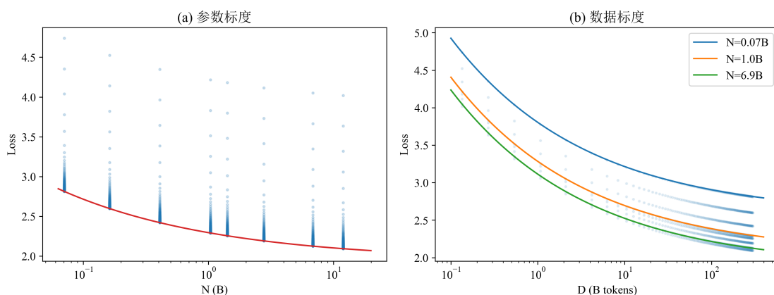
图 9 经典标度律对 Pythia 训练轨迹的拟合（左：随参数规模；右：随数据规模）
