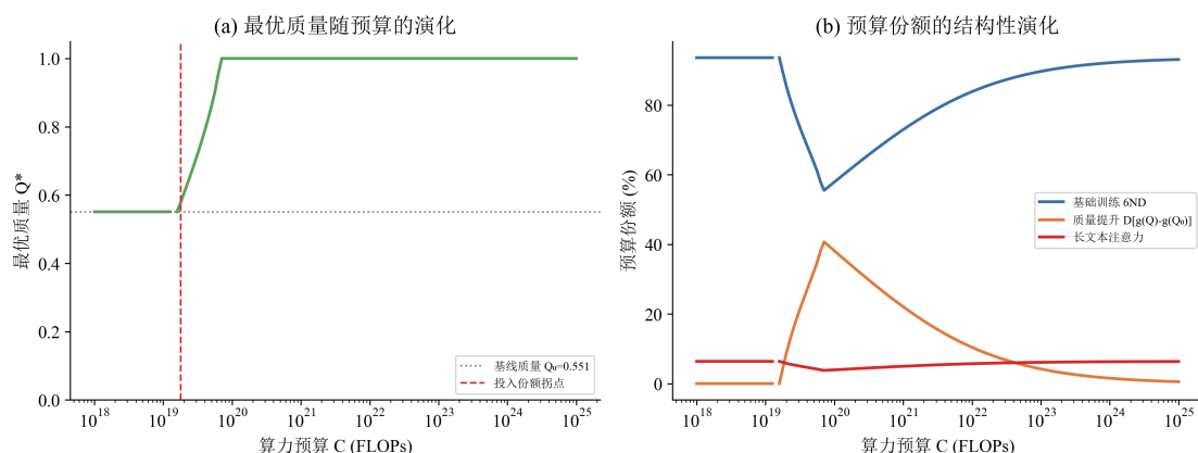
图 17 预算扫略下的资源配置结构性转移（左：最优质量演化；右：预算份额演化）
