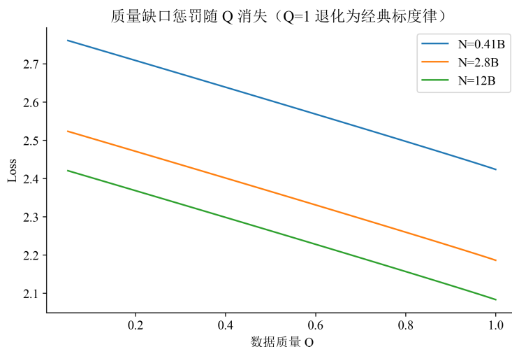
图 10 固定 N 、 D 时数据质量对损失的决定作用 ( Q = 1 退化为经典标度律)
