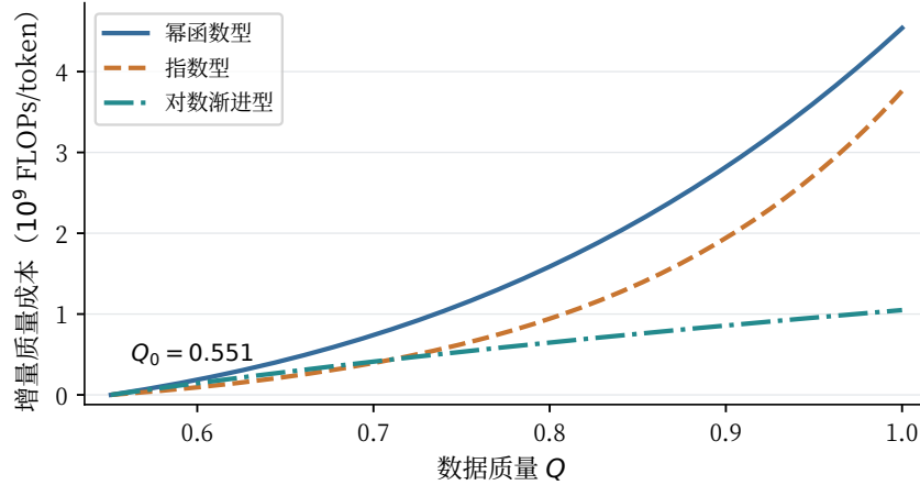
图 18 三类单位 token 增量质量成本 g(Q) - g(Q_0) （基线 Q_0 = 0.5510 ）。各曲线均从零增量成本出发，函数形式与系数见式(23)。
