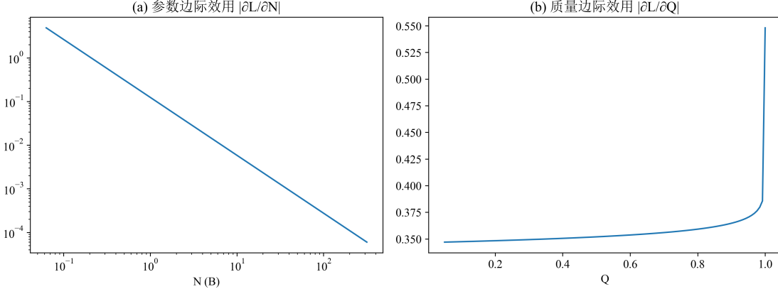
图 12 规模与质量的边际效应（左：随 N 衰减；右：在 Q < 1 内随 Q 缓慢增加）
