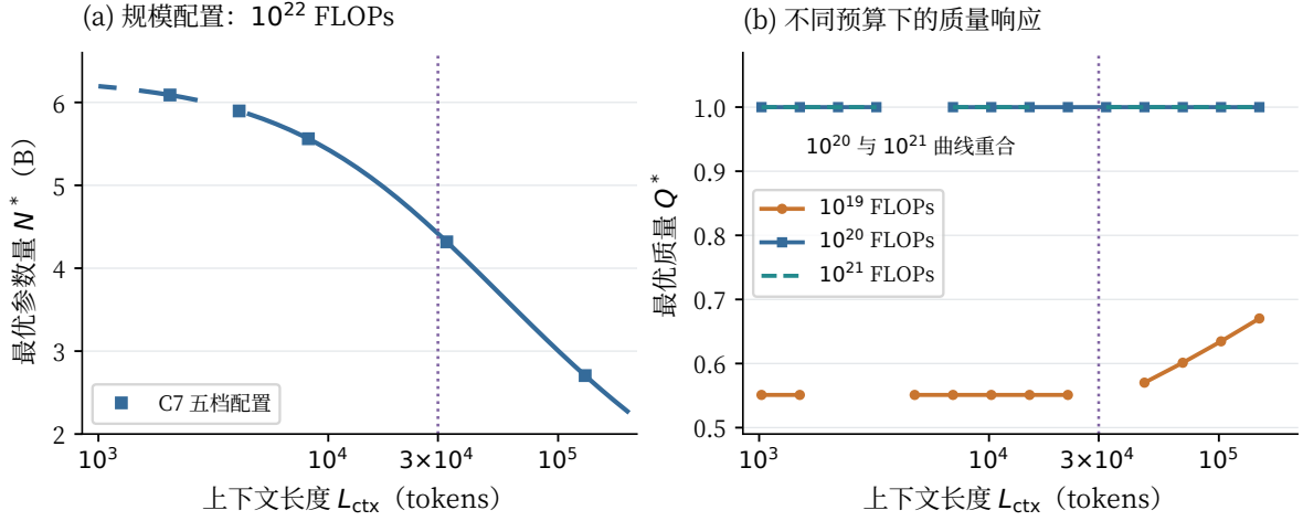
图 17 上下文长度对资源配置的影响（幂函数型成本， M = 0 ）。左： 10^{22} FLOPs 下的参数规模，方形点为 C7 五档配置；右： 10^{19} 、 10^{20} 、 10^{21} FLOPs 下的质量水平，后两条曲线重合。竖线表示注意力与基础训练成本相等的位置。
