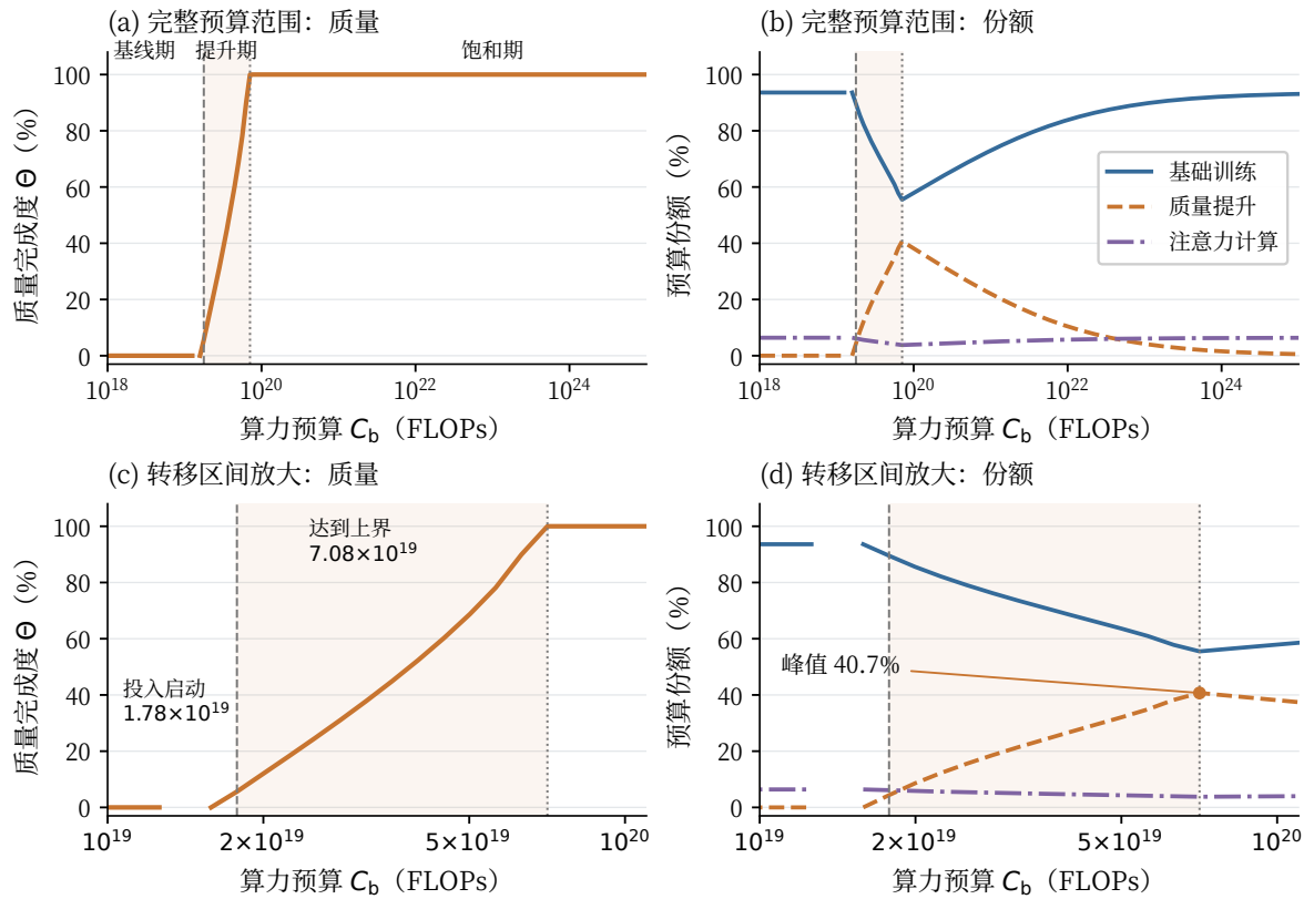
图 16 预算变化下的配置阶段 (幂函数型成本, L_{\text{ctx}} = 2048 , M = 0 )。上排为完整预算范围, 下排放大转移区间; 虚线表示首次观察到质量投入和饱和配置的网格预算, 曲线缺口对应求解失败点。
