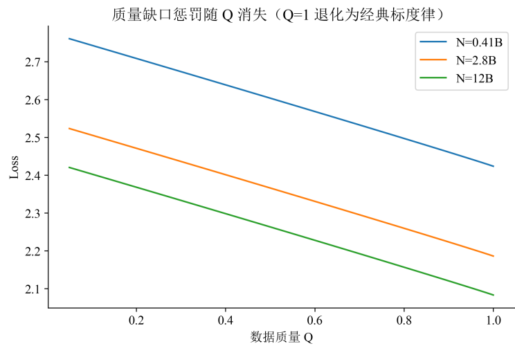
图 10 固定 N 、 D 时模型预测的质量效应 ( Q = 1 退化为经典标度律)
