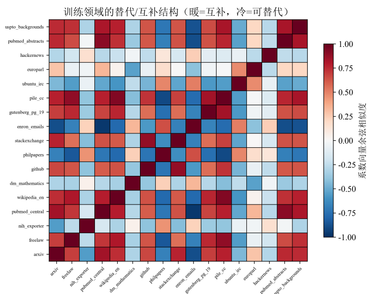
图 14 训练领域效应的余弦相似度（暖色为正、冷色为负；不直接表示互补增益）
