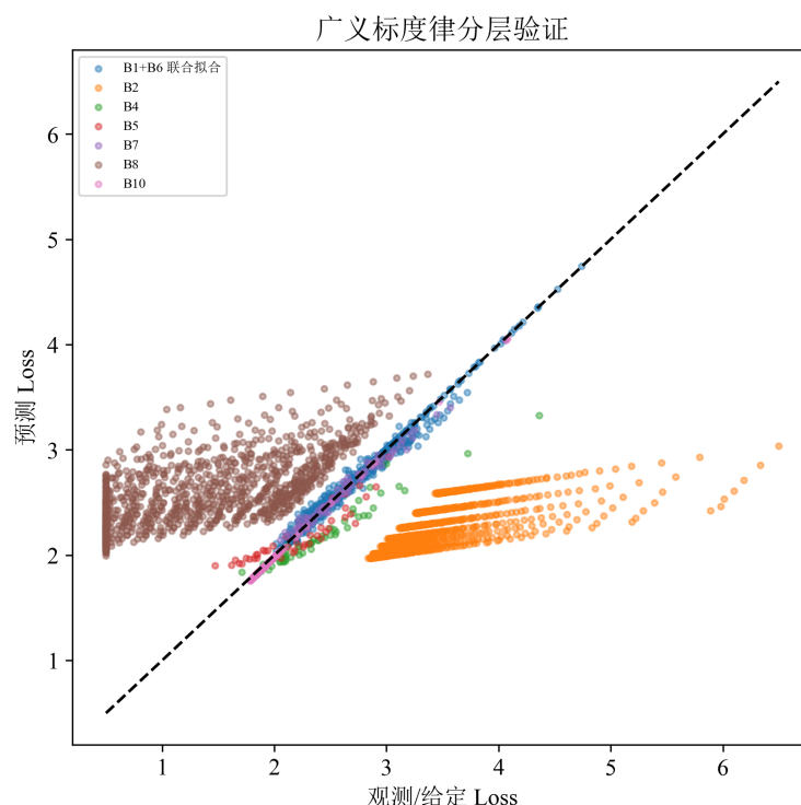
图 11 广义标度律预测值与给定损失的多源对比（含真实、半合成与估算数据）
