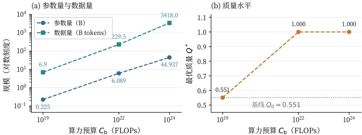
图 15 三档预算下的规模与质量配置。横轴按真实预算的对数间距排列；各点表示独立情景，虚线仅辅助比较。
