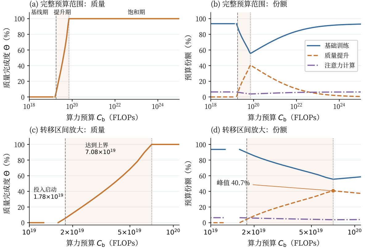
图 18 预算变化下的配置阶段（幂函数型成本， L_{\text{ctx}} = 2048 ， M = 0 ）。上排为完整预算范围，下排放大转移区间；虚线表示首次观察到质量投入和饱和配置的网格预算，曲线缺口对应求解失败点。
