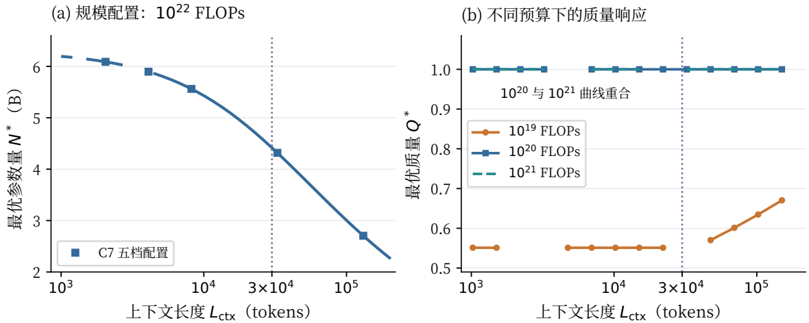
图 19 上下文长度对资源配置的影响 (幂函数型成本, M = 0 )。左: 10^{22} FLOPs 下的参数规模, 方形点为 C7 五档配置; 右: 10^{19} 、 10^{20} 、 10^{21} FLOPs 下的质量水平, 后两条曲线重合。竖线表示注意力与基础训练成本相等的位置。
