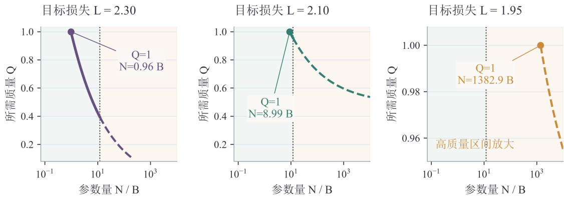
D=300B tokens；实线： N \leq 12B ；虚线：规模外推。 右图纵轴单独放大；阴影区分拟合规模与外推规模。
