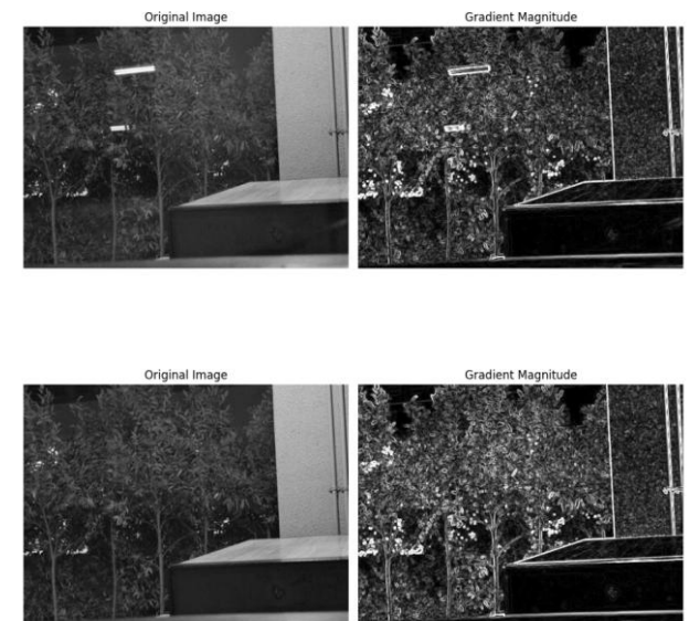
圖 4. Sobel 梯度幅度視覺化(左:原始影像;右:梯度幅度圖)。上:含反光場景——反光區僅在邊界產生高梯度、內部梯度低;下:無反光場景——梯度集中於物件結構邊緣。此對比即 SGA 注意力引導信號的 domain-agnostic 物理基礎。
