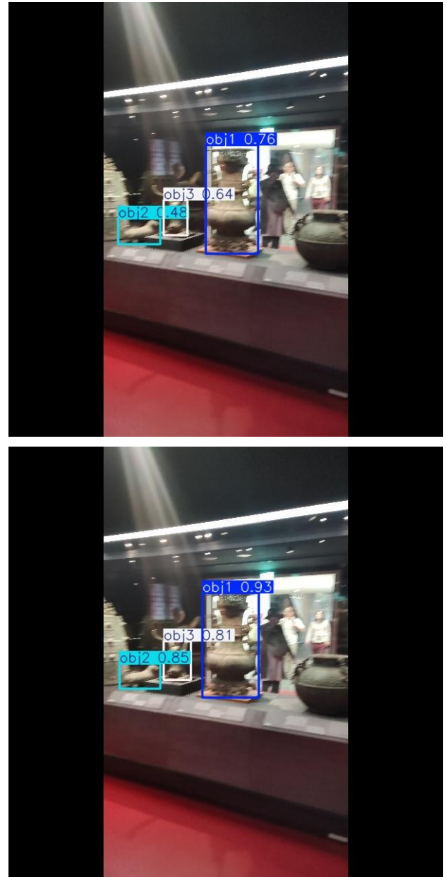
圖 6. YOLOv8 辨識結果範例：原始含反光影像（上）與 Pix2Pix+SGA 處理後影像（下）之偵測框與信心值比較。三個物件的辨識信心值分別由 0.76、0.48、0.64 提升至 0.93、0.85、0.81。
