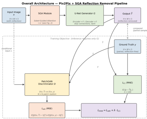
圖 1. 整體架構示意圖。輸入影像 x (含反光) 經 SGA 模組 (結構詳見圖 2) 重校準為 x' ，再由 U-Net 生成器 G (Encoder \times 7 / Decoder \times 7 ，含 skip connection, tanh 輸出) 映射為去反光輸出 T^* 。訓練階段另以 PatchGAN 判別器 D 比較 (x, T^*) 與 (x, y) 計算對抗損失 L_{adv} ，並將 T^* 與 ground truth y 比較計算 L_{L1} ，合併為 L_{total} = L_{adv} + \lambda \cdot L_{L1} ( \lambda = 100 )；推論階段僅需生成器 G 。
