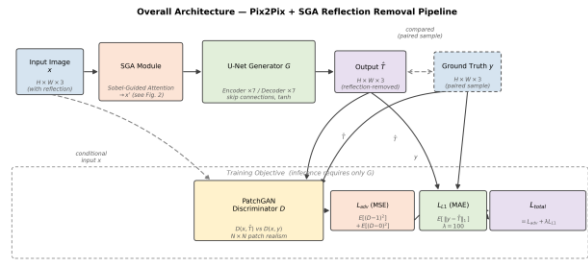
圖 1. 整體架構示意圖。輸入影像 x (含反光) 經 SGA 模組 (結構詳見圖 2) 重校準為 x' ，再由 U-Net 生成器 G (Encoder \times 7 / Decoder \times 7 ，含 skip connection, tanh 輸出) 映射為去反光輸出 T^{\wedge} 。訓練階段另以 PatchGAN 判別器 D 比較 (x, T^{\wedge}) 與 (x, y) 計算對抗損失 L_{adv} ，並將 T^{\wedge} 與 ground truth y 比較計算 L_{L1} ，合併為 L_{total} = L_{adv} + \lambda \cdot L_{L1} ( \lambda = 100 )；推論階段僅需生成器 G 。
