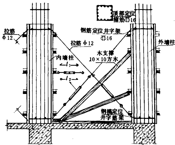
图3 柱模找正方法示意
