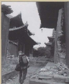
报恩寺背后山墙倒塌，山门口左侧的哈将塑像手臂、腿、脚等处不同程度受损。
