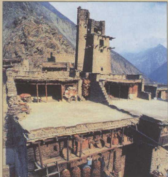
在理县桃坪羌寨，体现羌族高超建筑艺术的碉楼受损严重。
