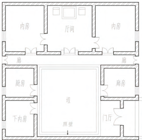
图2 雷州三合院平面布局（图片来源：作者自绘）
