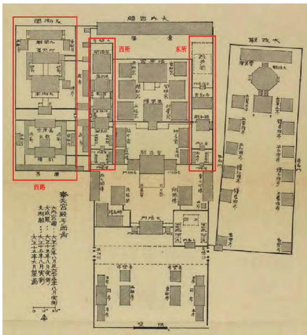
图2 伊藤清造《奉天宫殿建筑图集》中的沈阳宫殿平面图 （作者添绘）
