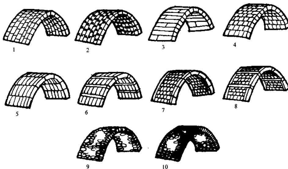
图 3.10 中国石拱拱券砌筑方式
