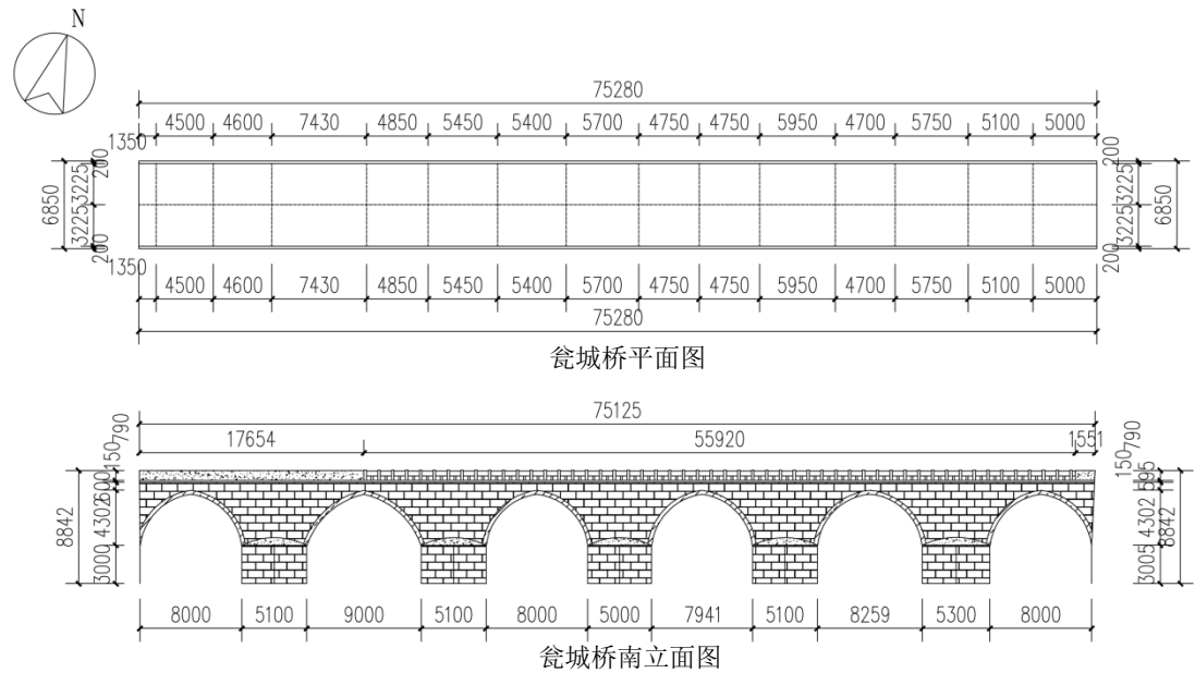
图 2.14 贵定县盘江镇瓮城桥南立面图和平面图 作者自绘
