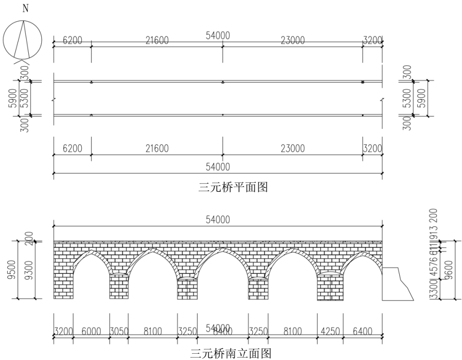
图 2.8 龙里县三元镇三元桥平面图和南立面图 作者自绘
