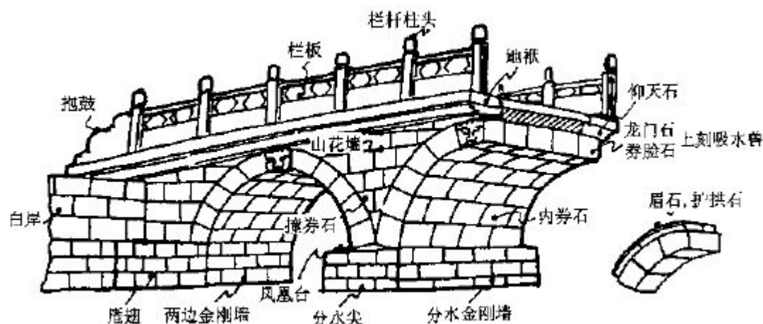
图 3.1 清·官式石拱桥各部名称图
