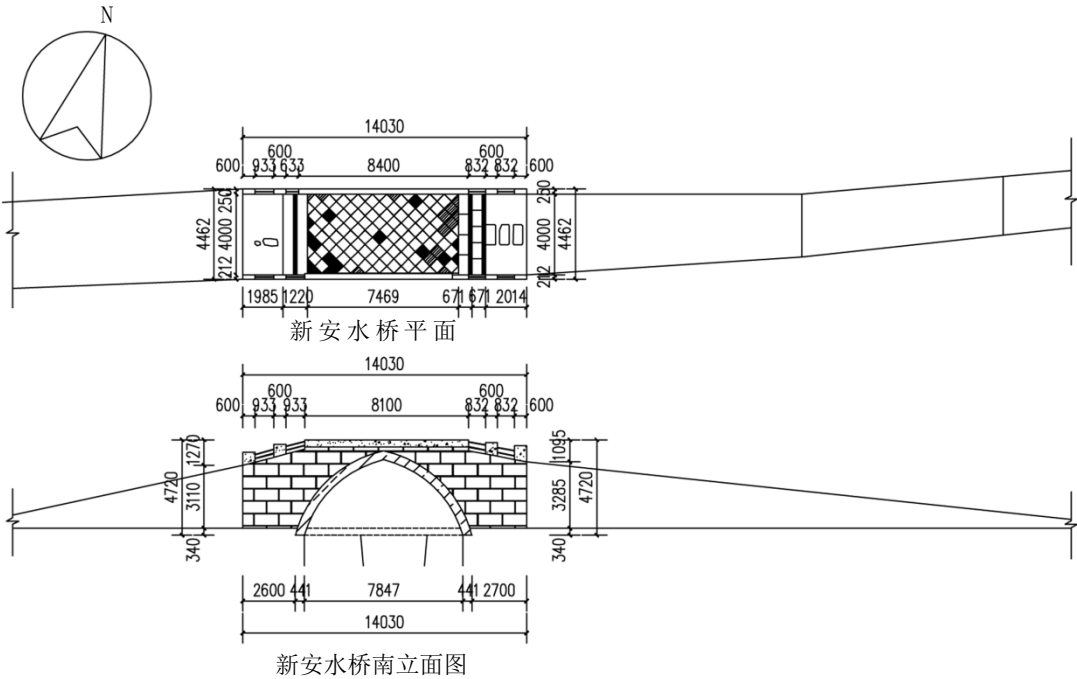
图 2.11 龙里县三元镇新安村新安水桥平面图和南立面图 作者自绘
