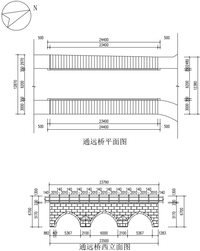
图 2.19 福泉市通远桥平面图和西立面图 作者自绘
