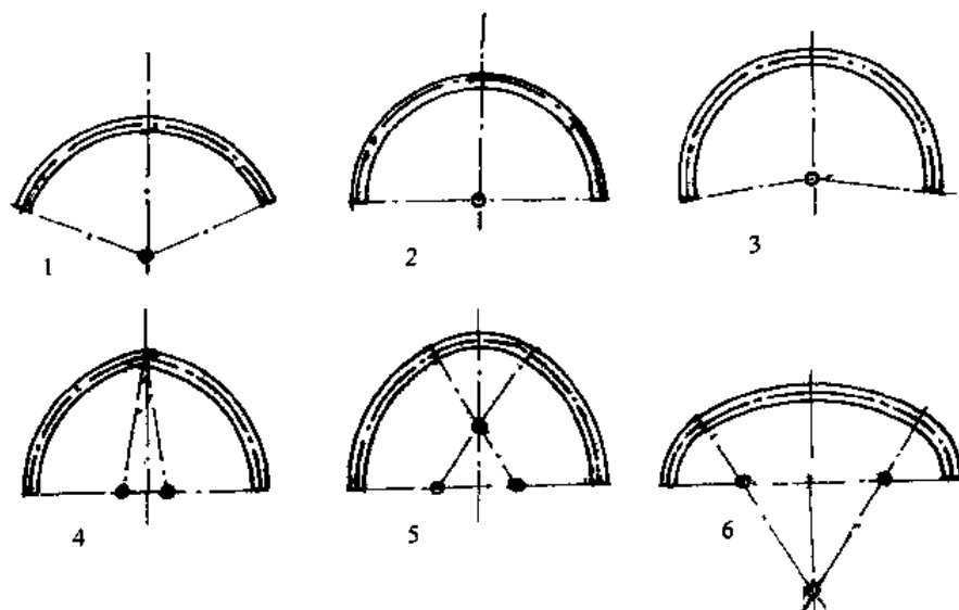
图 3.9 中国石拱拱券各种拱轴线
