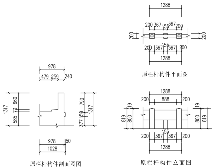
图 2.15 贵定县盘江镇瓮城桥细部构件 作者自绘
