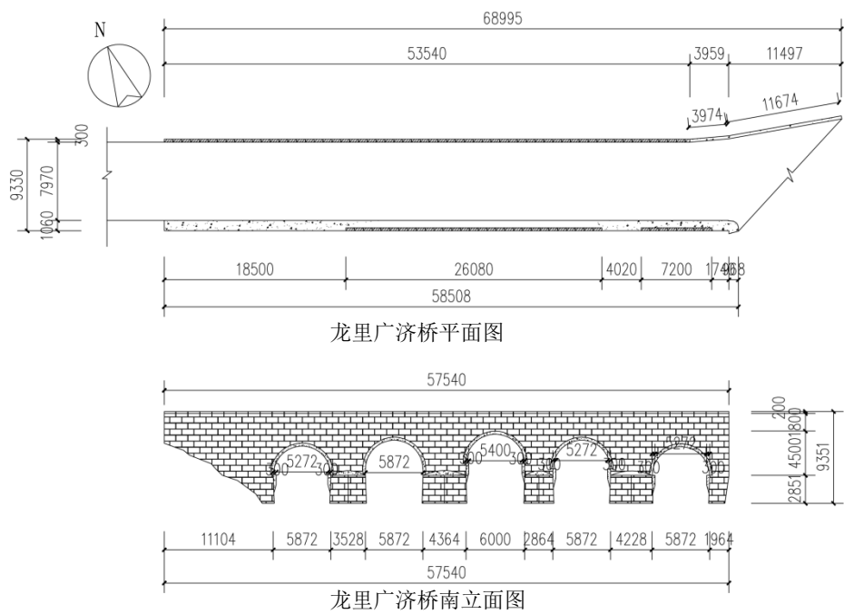
图 2.6 龙里广济桥平面图及南立面图 作者自绘
