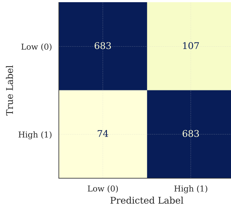
ET (Original)
