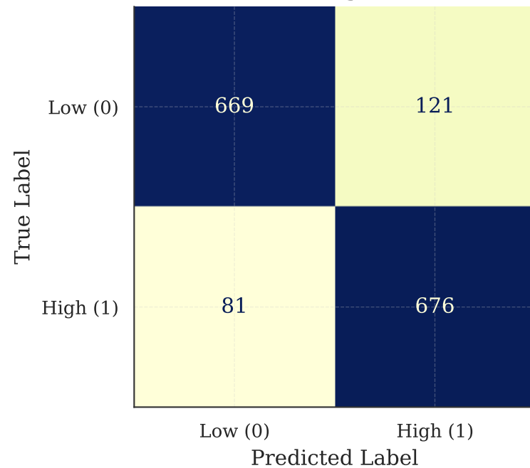
ET (Original)
