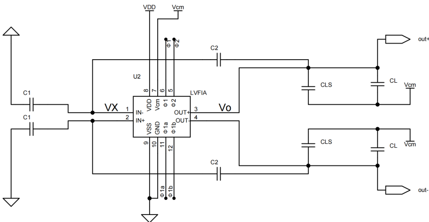
图 3.3 初步放大时的电路连接关系
