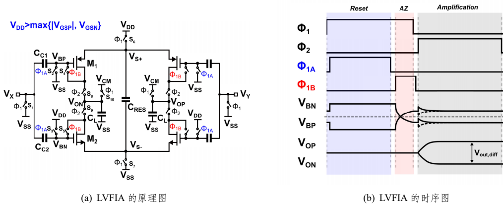
图 2.4 LVFIA 的原理图和时序图
