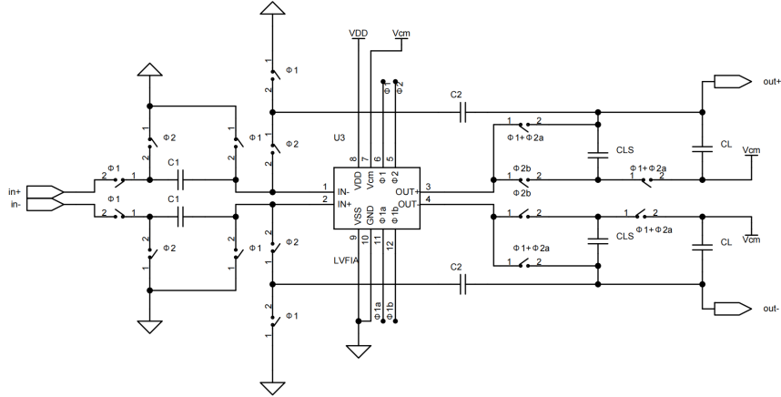
图 3.1 本论文所提出的基于 LVFIA 和 CLS 机制的动态放大器设计
