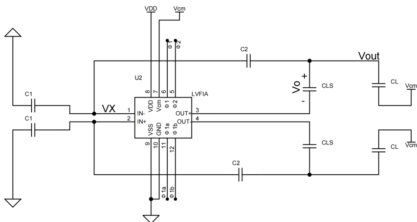
图 3.4 电平移位时的电路连接关系
