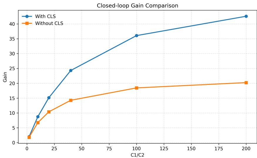
图 4.4 闭环增益随 C_1/C_2 变化的趋势图
