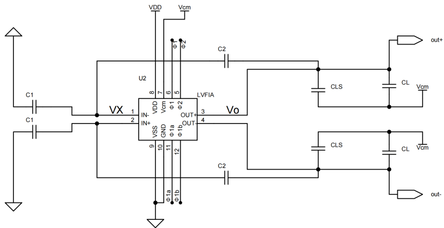
图 3.3 初步放大时的电路连接关系
