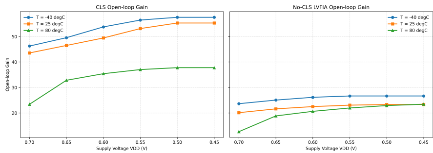
图 4.3 开环增益随 PVT 变化的趋势图
