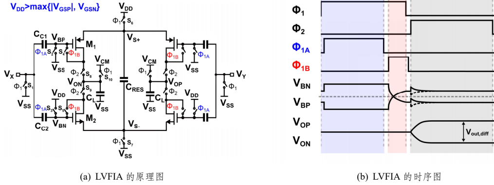
图 2.4 LVFIA 的原理图和时序图
