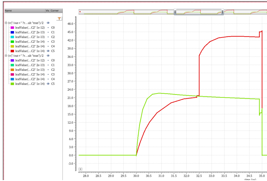
图 4.5 有无 CLS 下的瞬态响应对比
