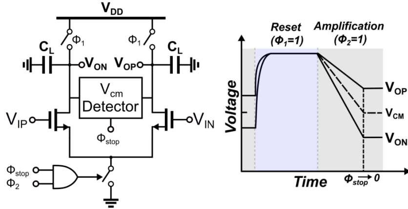
图 2.1 基本动态放大器的原理图和时序图
