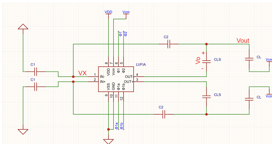
图 3.4 电平移位时的电路连接关系
