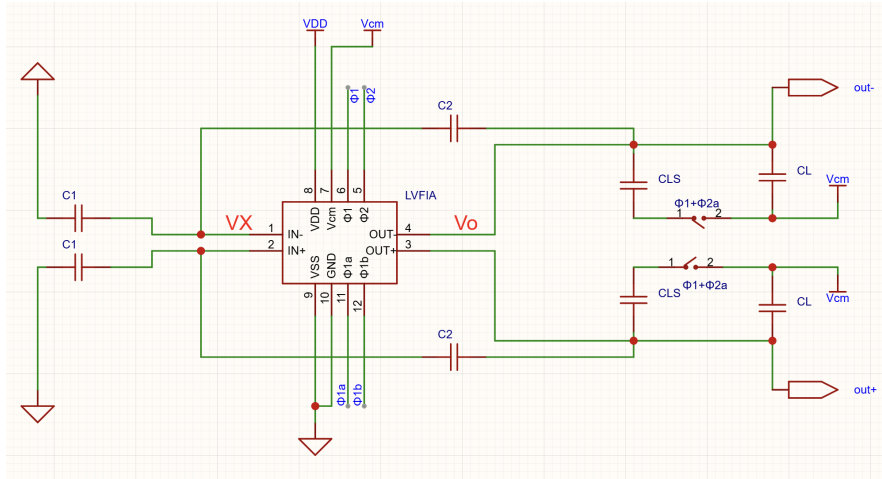
图 3.3 初步放大时的电路连接关系
