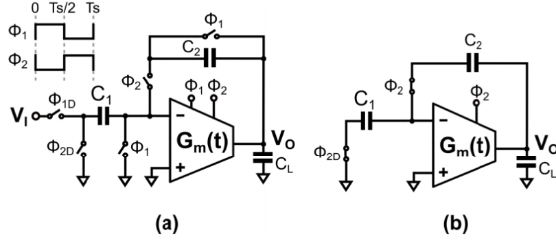
图 2.5 基于 LVFIA 的开关电容积分器电路设计
