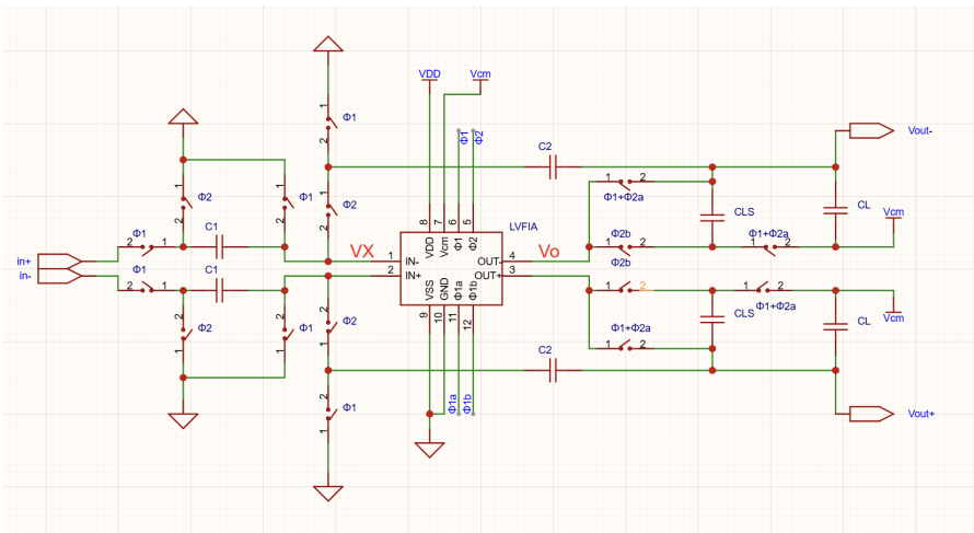
图 3.1 本论文所提出的基于 LVFIA 和 CLS 机制的动态放大器设计
