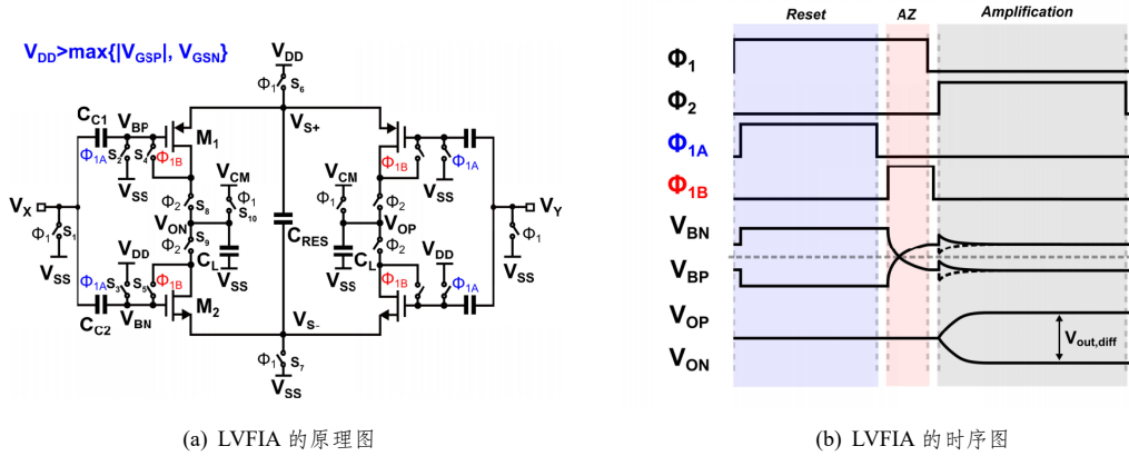
图 2.4 LVFIA 的原理图和时序图
