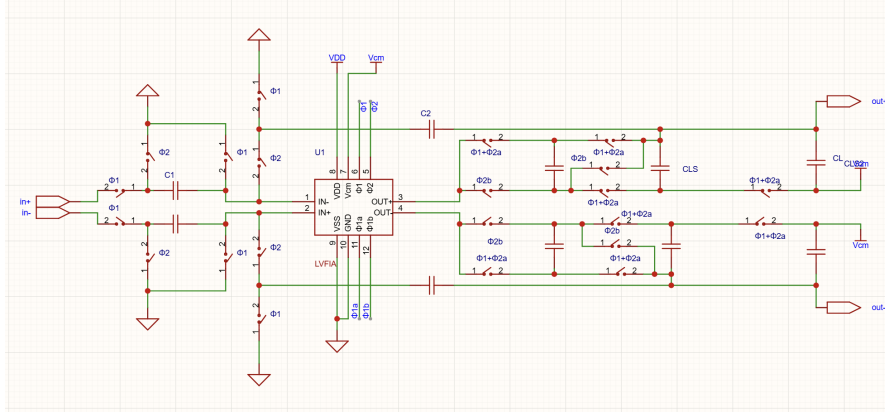
图 3.5 本论文所提出的基于 LVFIA 和 CLS 机制的动态放大器设计
