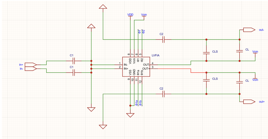
图 3.2 复位时的电路连接关系
