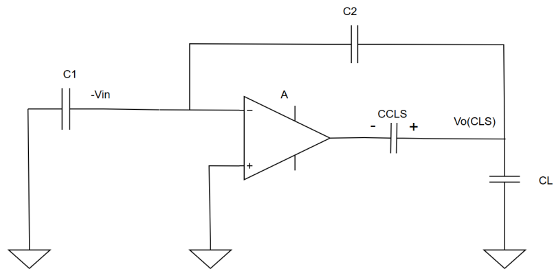
(b) CLS 电平移位阶段时的电路连接图
