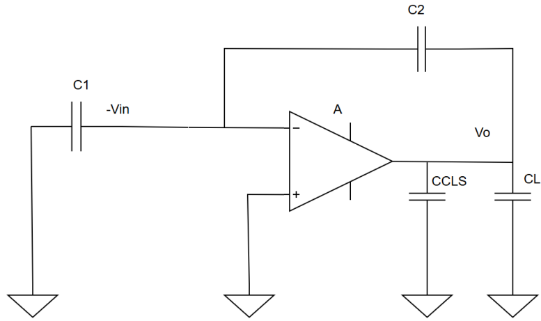
(a) CLS 初步放大阶段时的电路连接图
