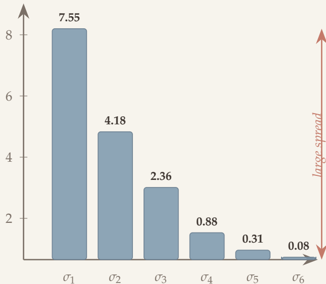
Gradient G: singular values
