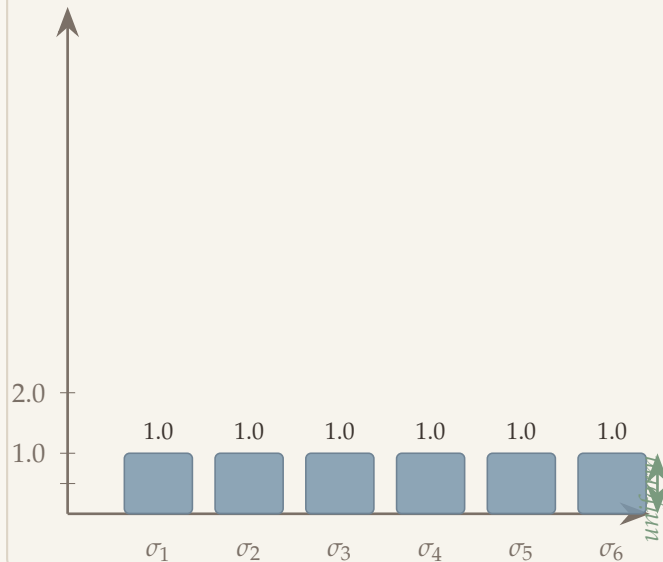
Muon update UV^\top : singular values
