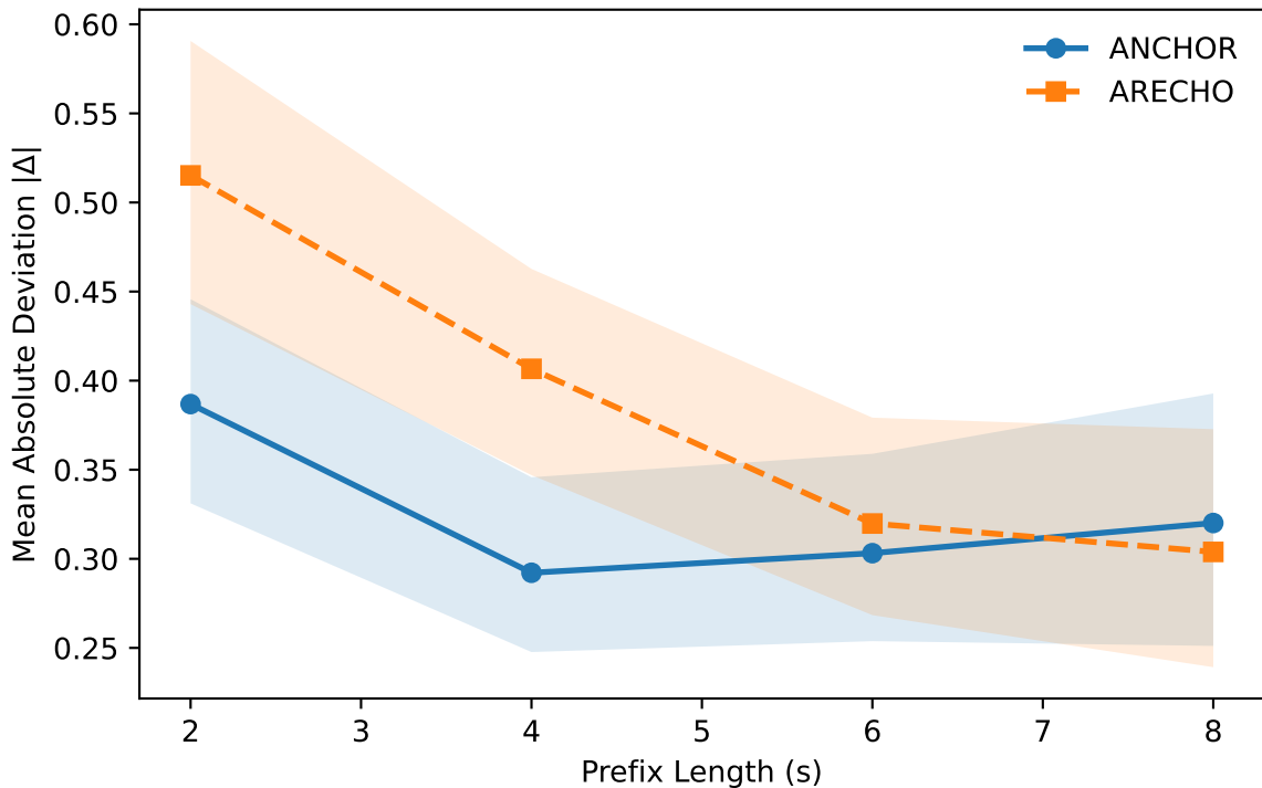
Robustness Curve — utmosv2
