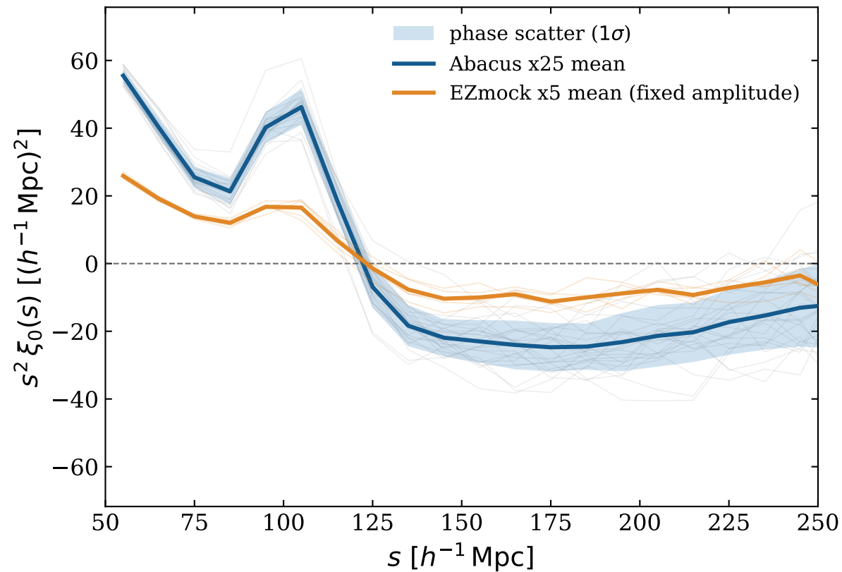
Periodic-box 2PCF
