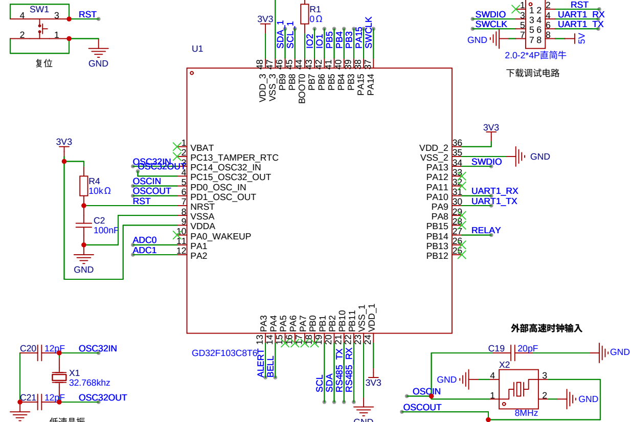
单片机系统电路
