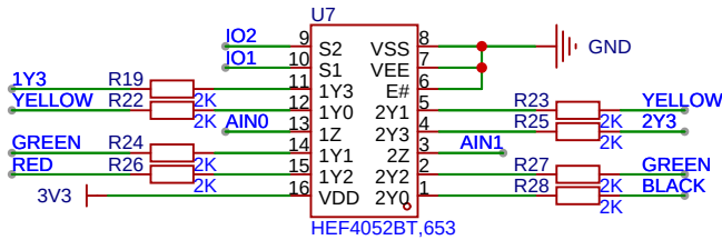
ADC检测电路
