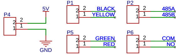
接线端子
