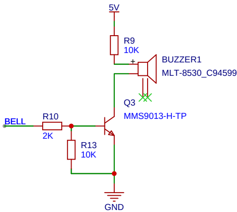
蜂鸣器驱动电路
