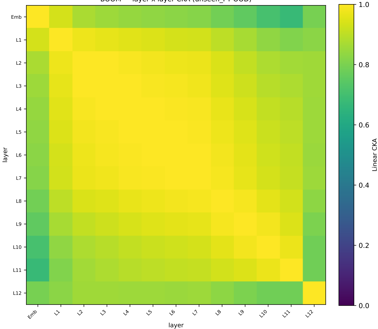
BOOM — layer x layer CKA (unseen_PT-OOD)
