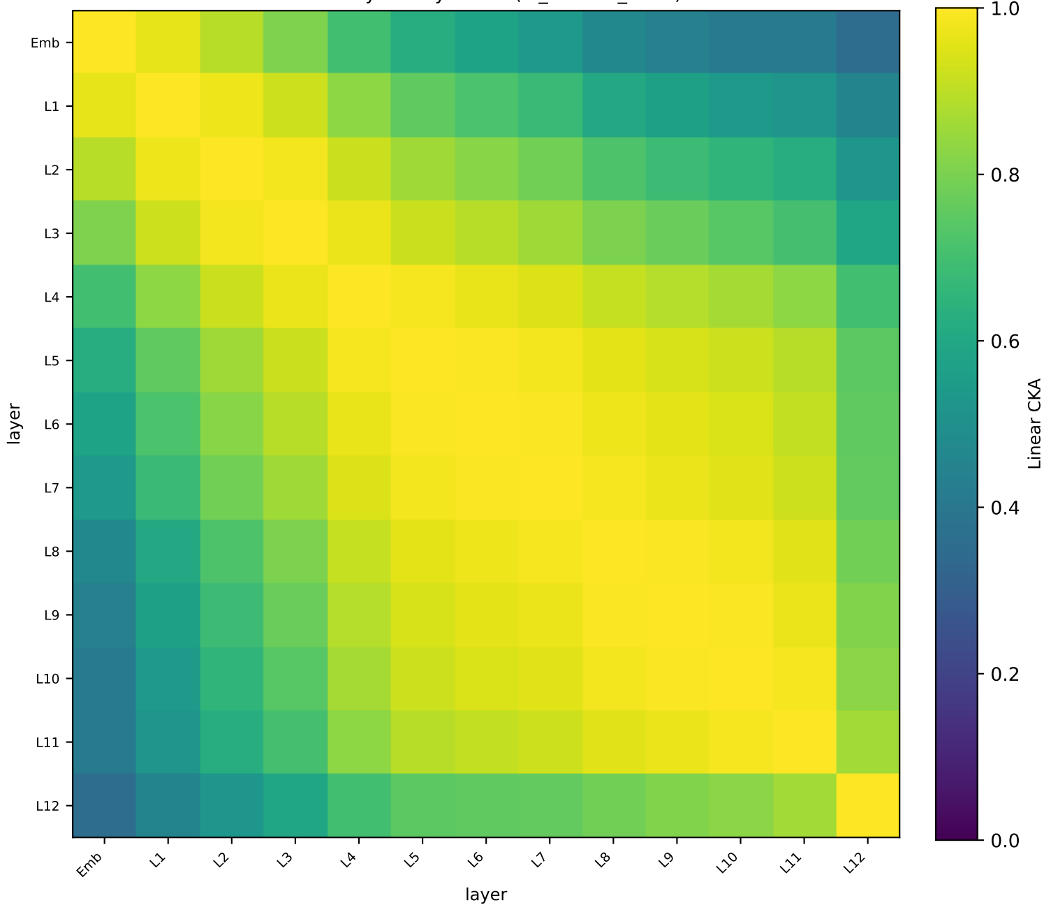
M4 — layer x layer CKA (in_domain_PT-ID)
