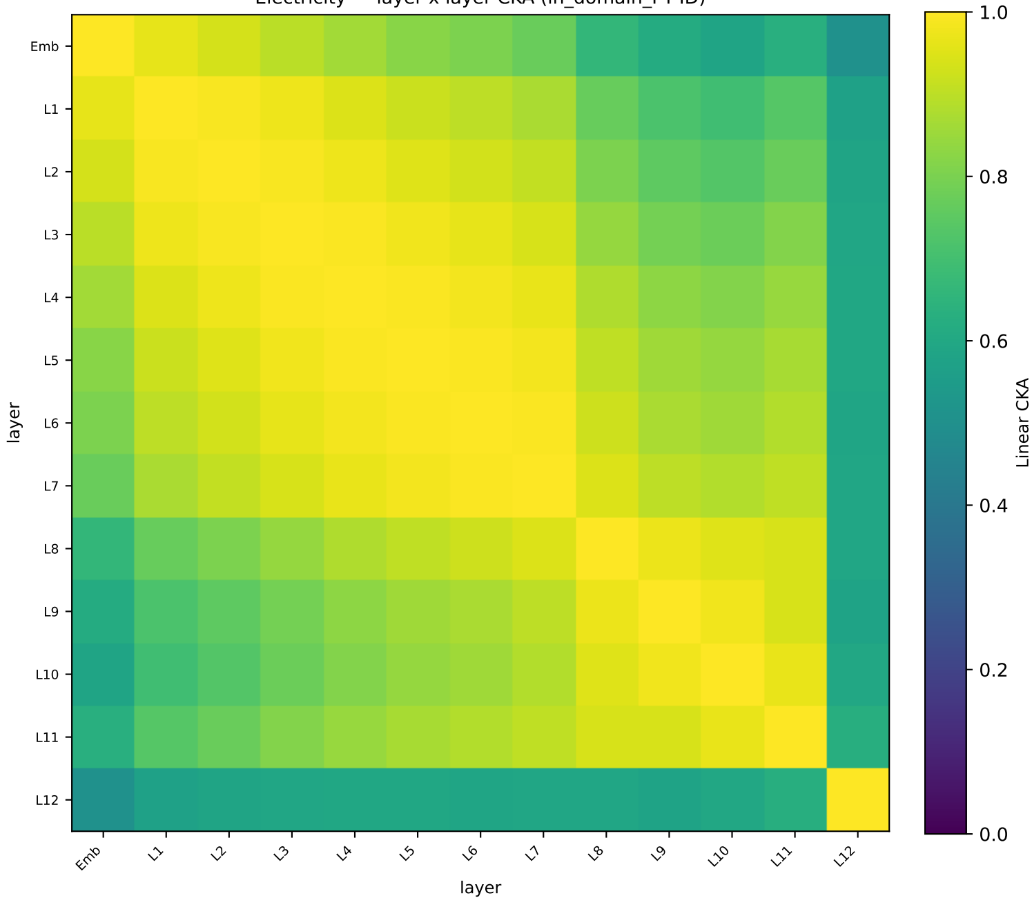
Electricity — layer x layer CKA (in_domain_PT-ID)
