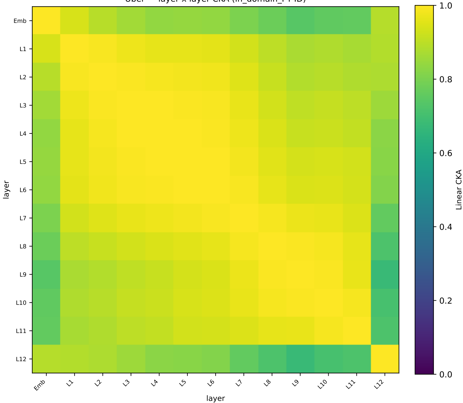
Uber — layer x layer CKA (in_domain_PT-ID)
