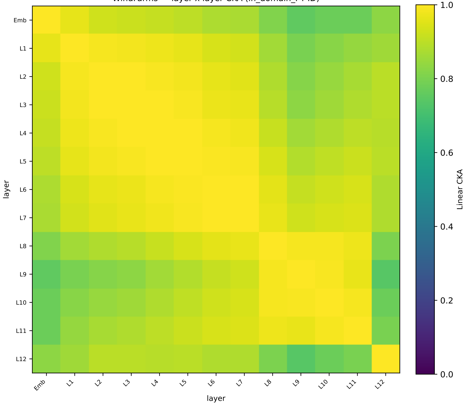
WindFarms — layer x layer CKA (in_domain_PT-ID)
