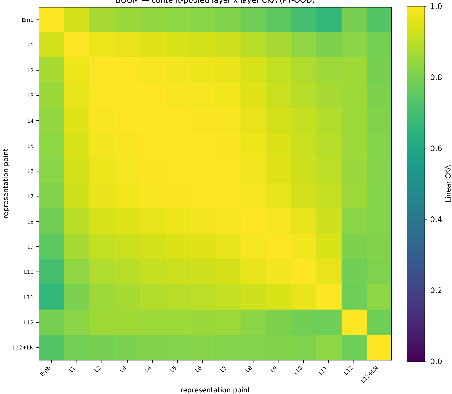
BOOM — content-pooled layer x layer CKA (PT-OOD)
