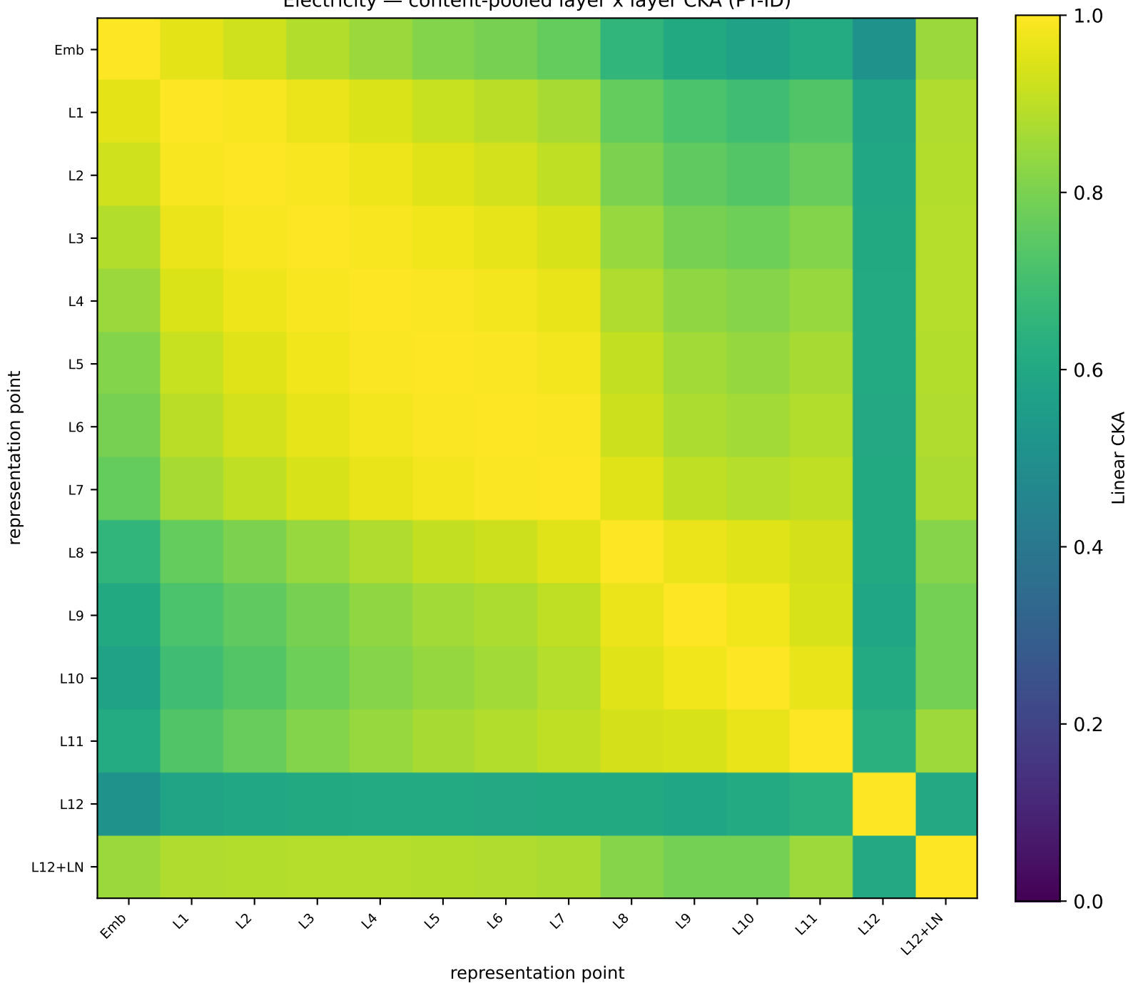
Electricity — content-pooled layer x layer CKA (PT-ID)
