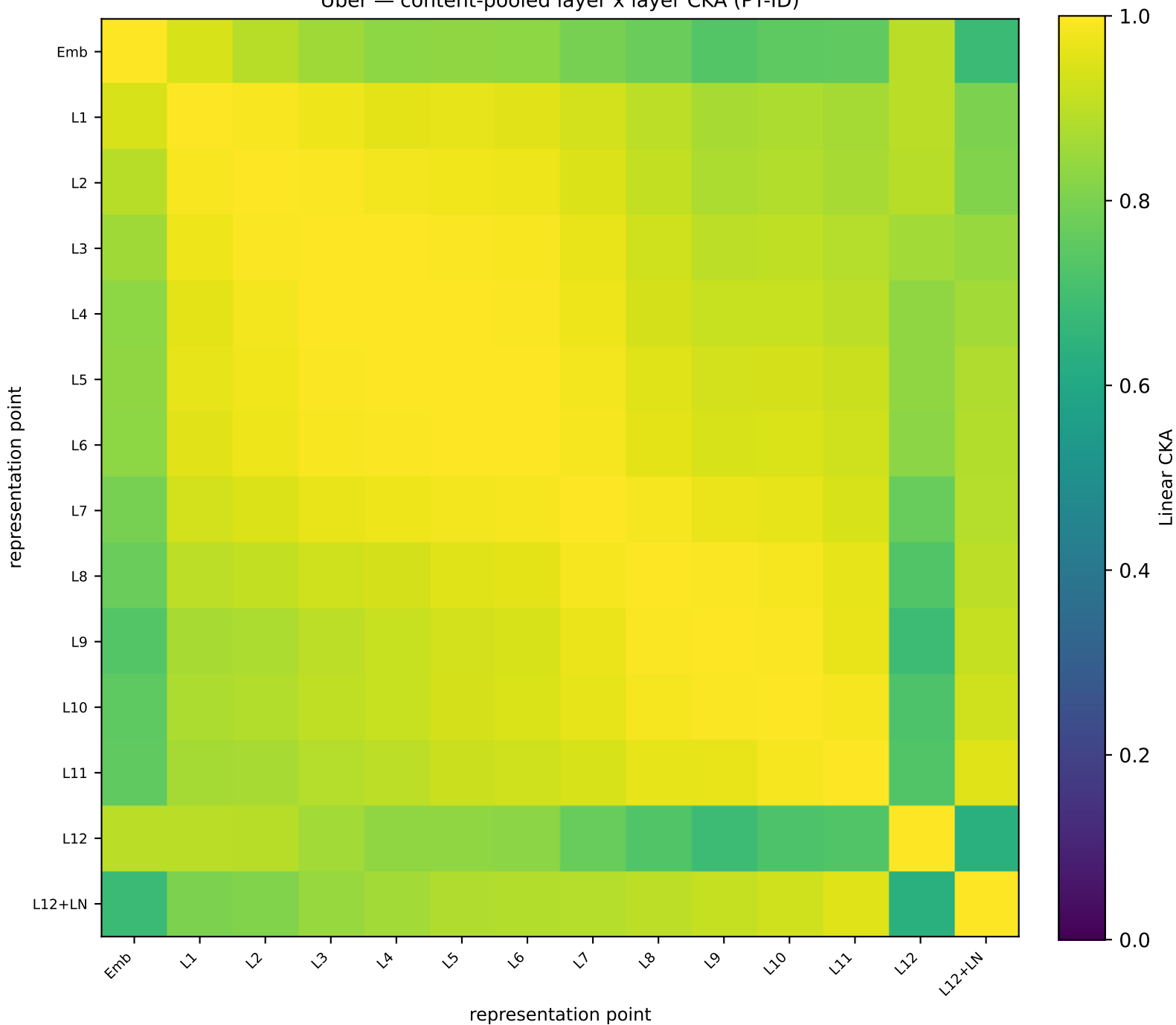
Uber — content-pooled layer x layer CKA (PT-ID)
